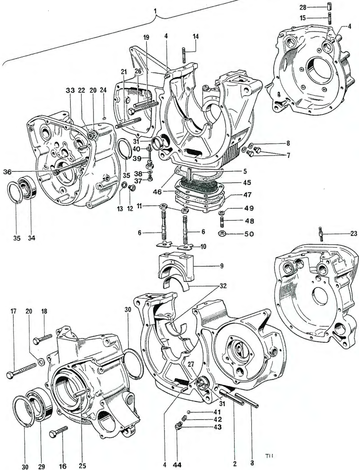
Fig. 2. CRANKCASES
