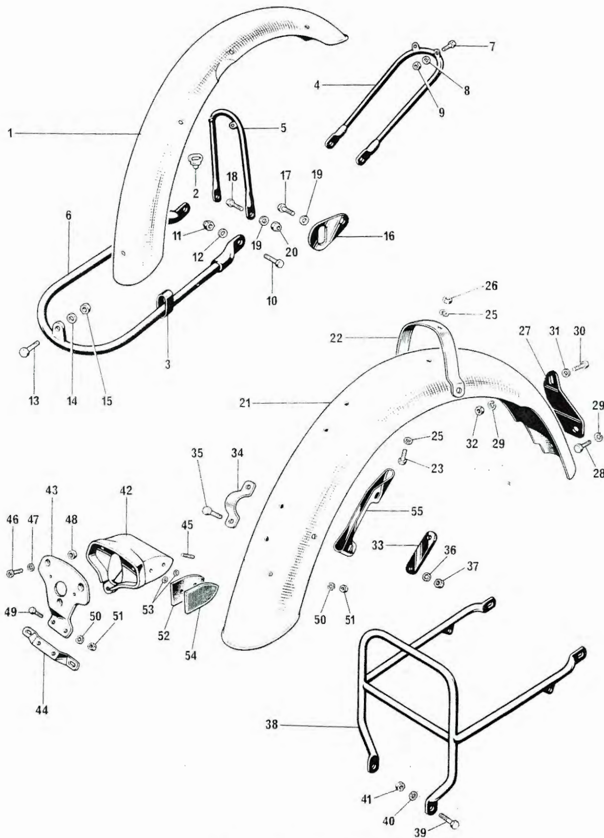
Fig. 27. MUDGUARDS (FENDERS)
