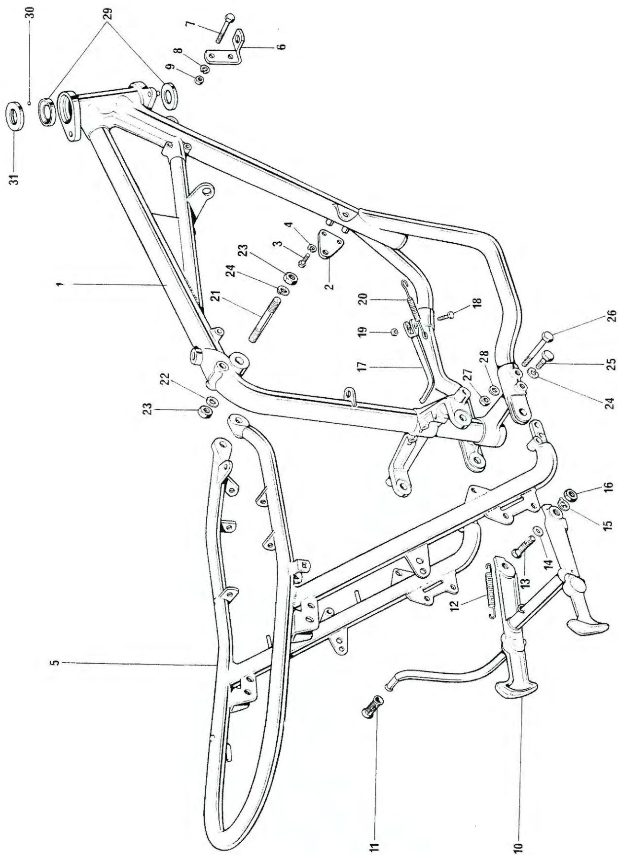
Fig. 14. FRAME
