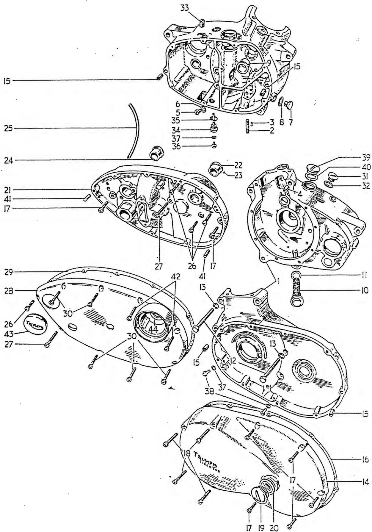
Fig. 2. CRANKCASE
