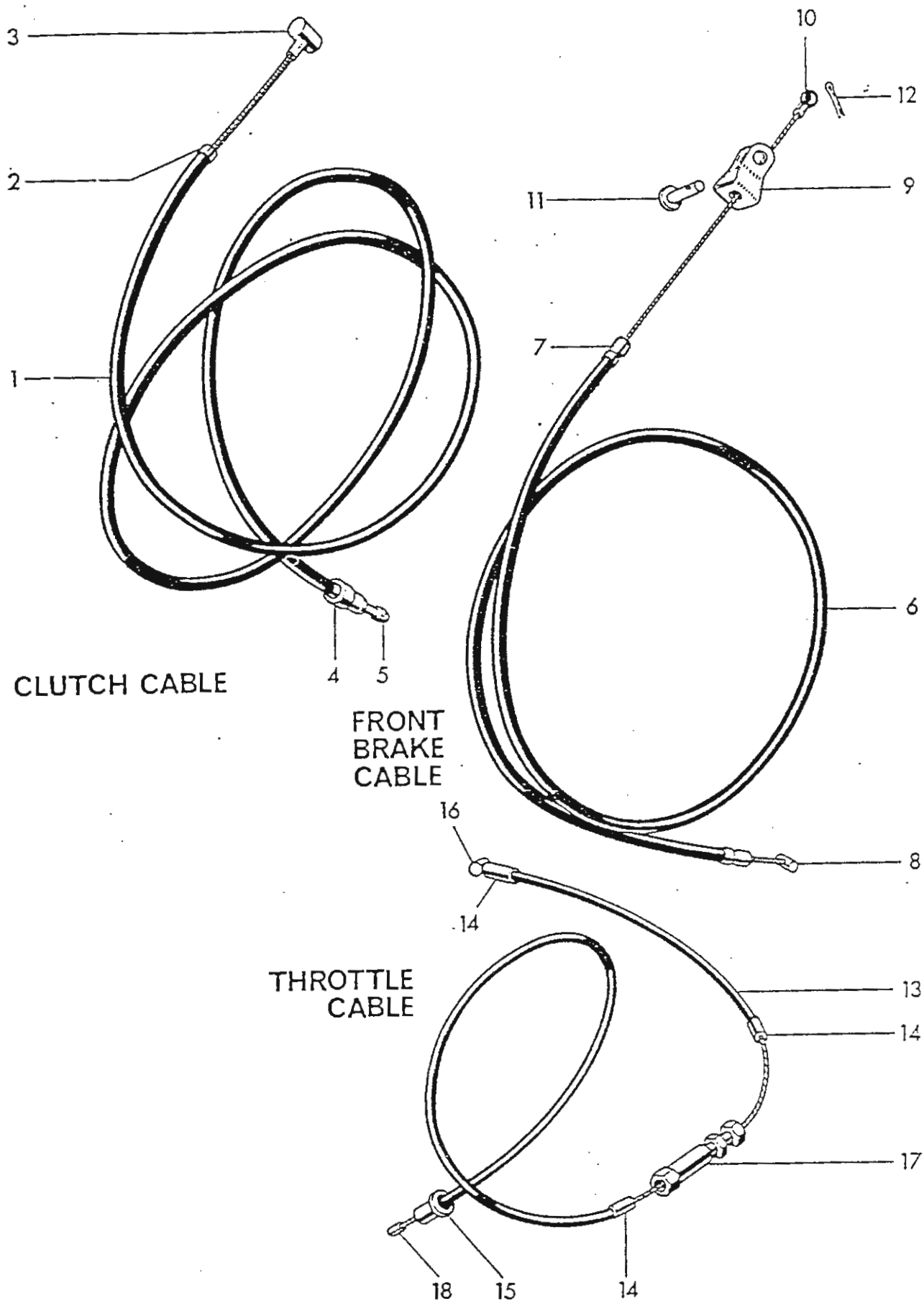
Fig. 17. CONTROL CABLES
