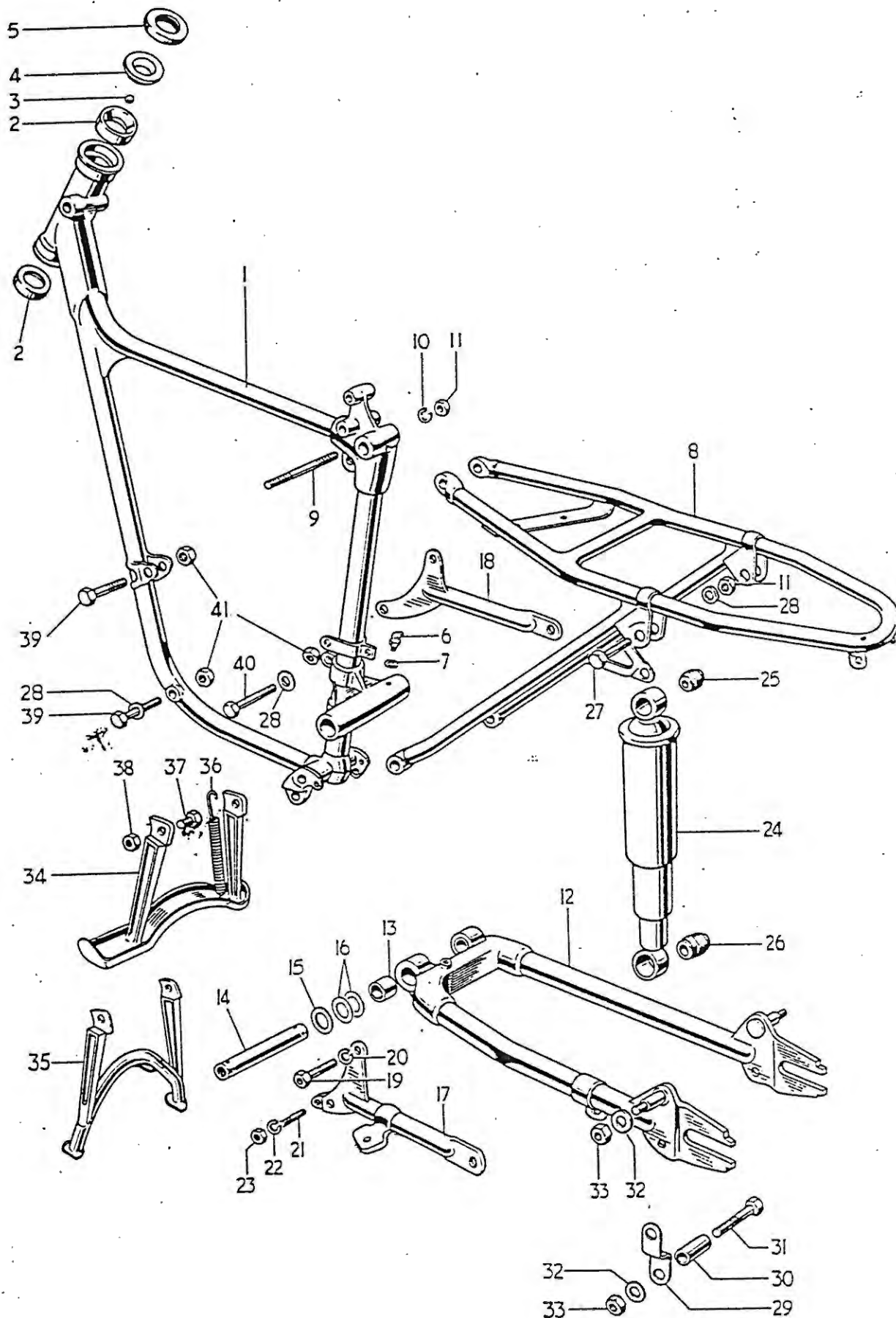
Fig. 7. FRAME COMPLETE
