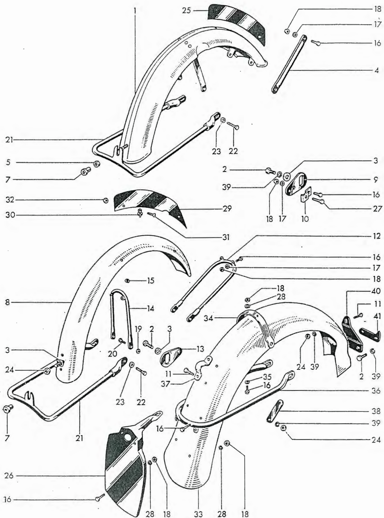
Fig. 26. MUDGUARDS
