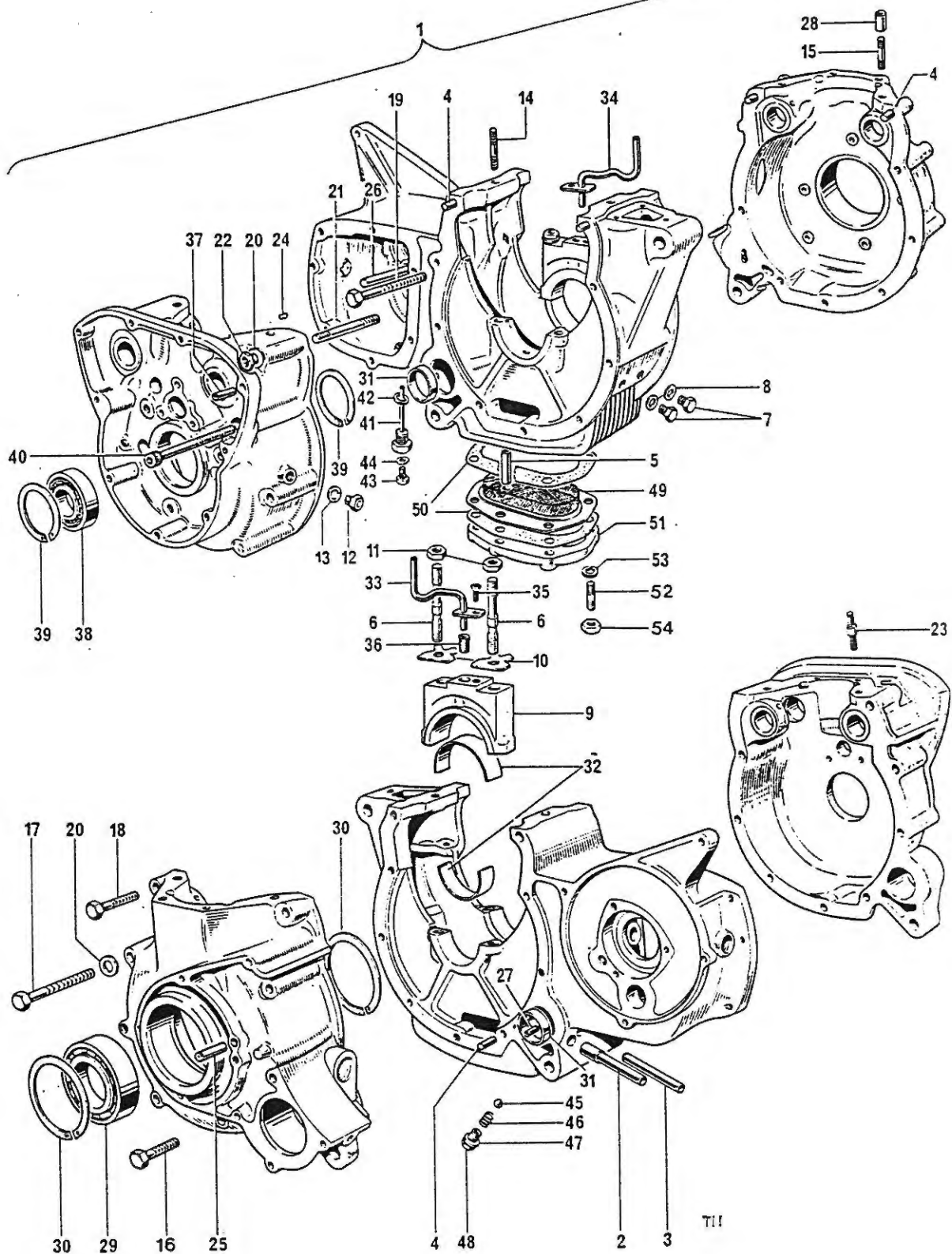
Fig. 2. CRANKCASES
