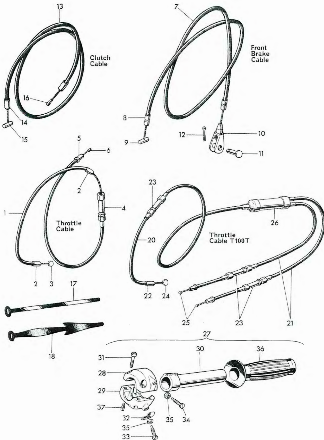
Fig. 28. CONTROL CABLES
