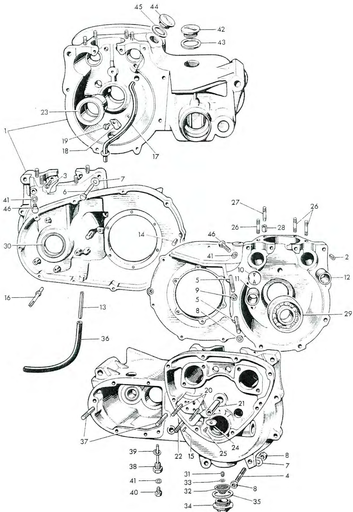
Fig. 2. CRANKCASE
