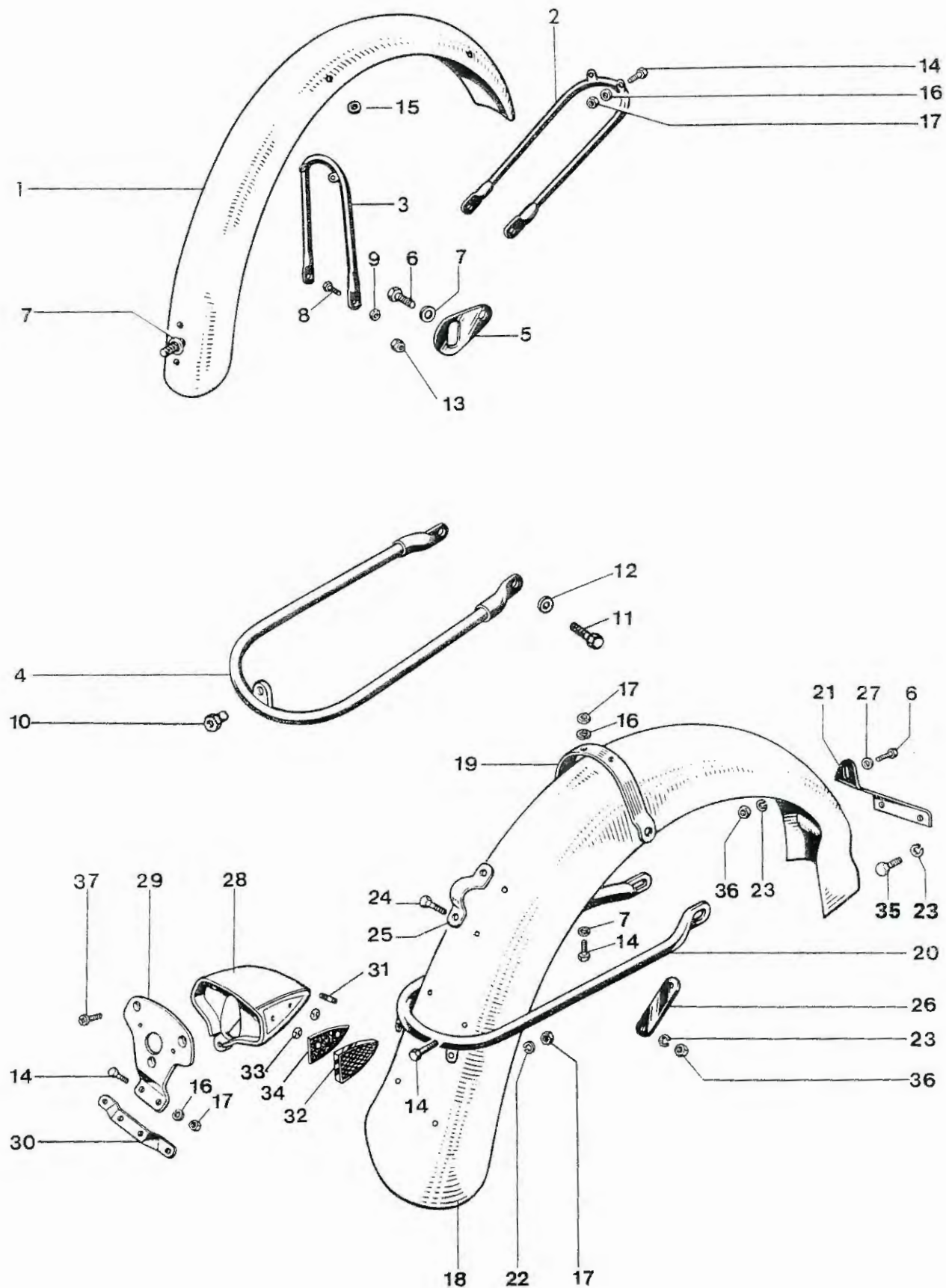
Fig. 26. FENDERS
