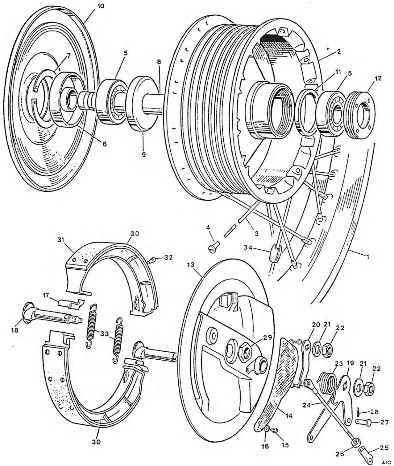
Fig. 10. FRONTWHEEL
