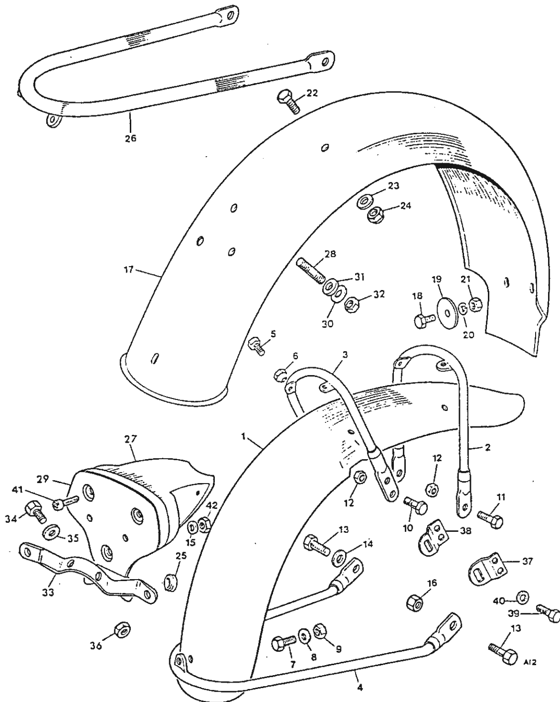
Fig. 12. FENDERS
