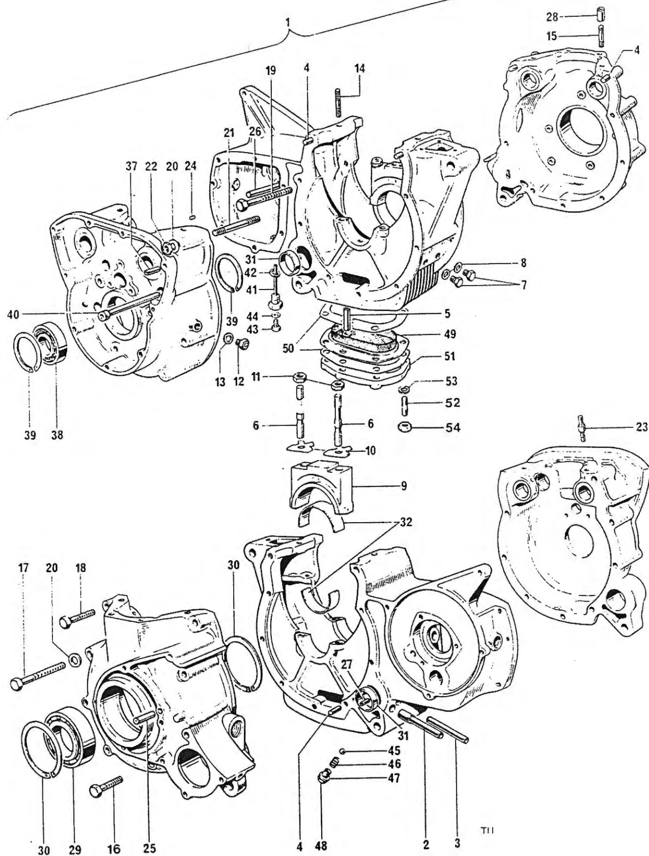
Fig. 2. CRANKCASES
