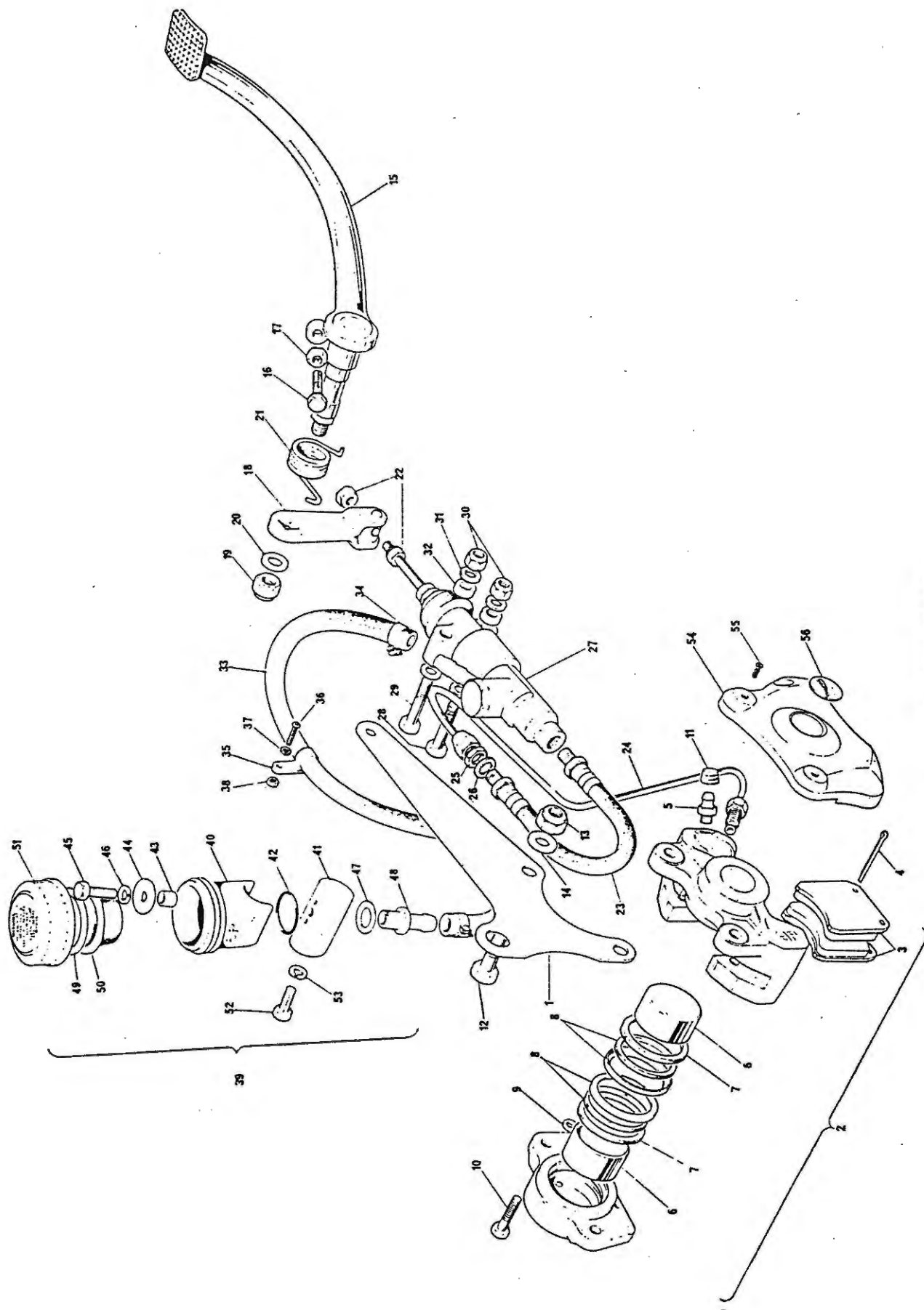
Fig. 25. REAR BRAKE
