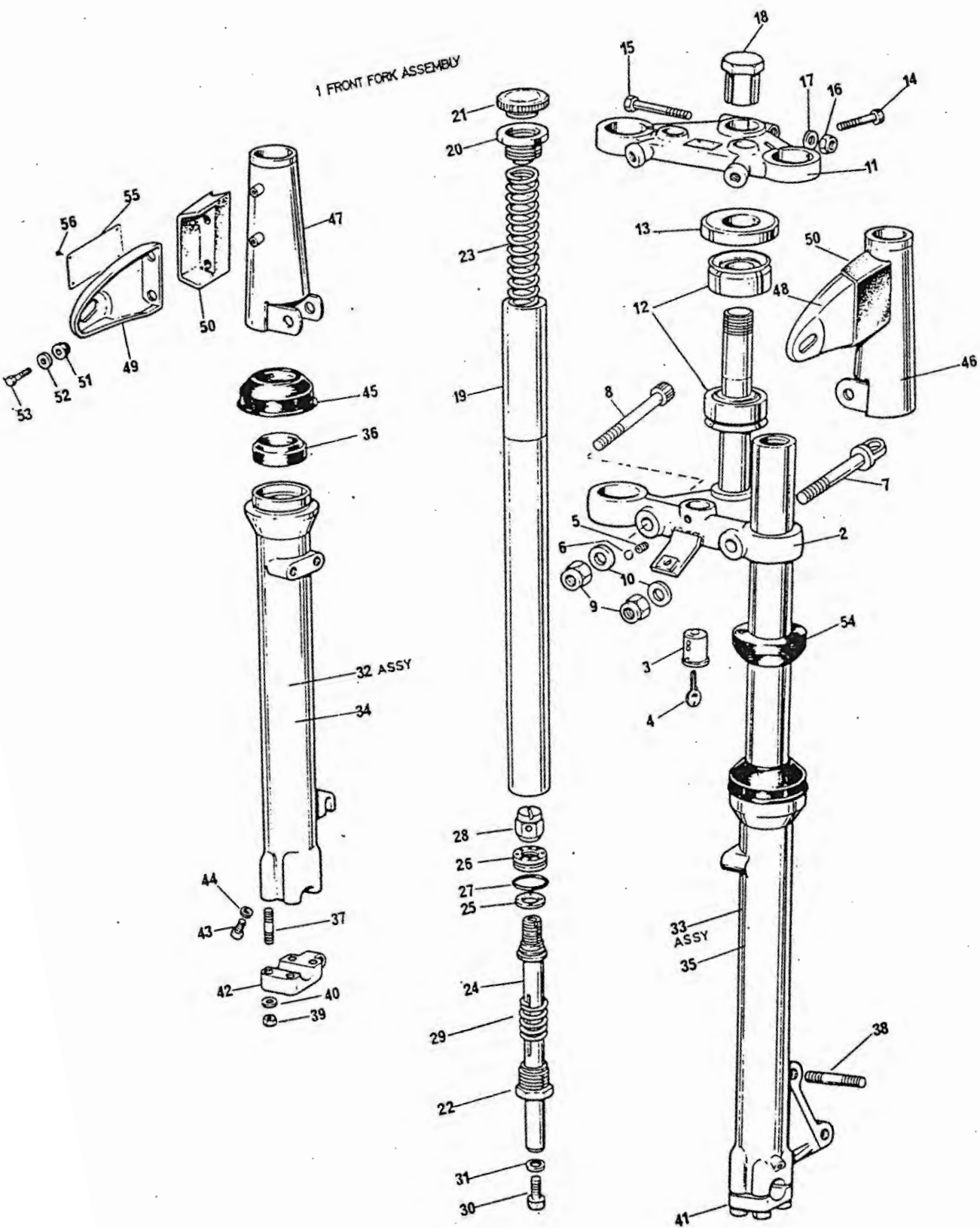
Fig. 21. FRONT FORK
