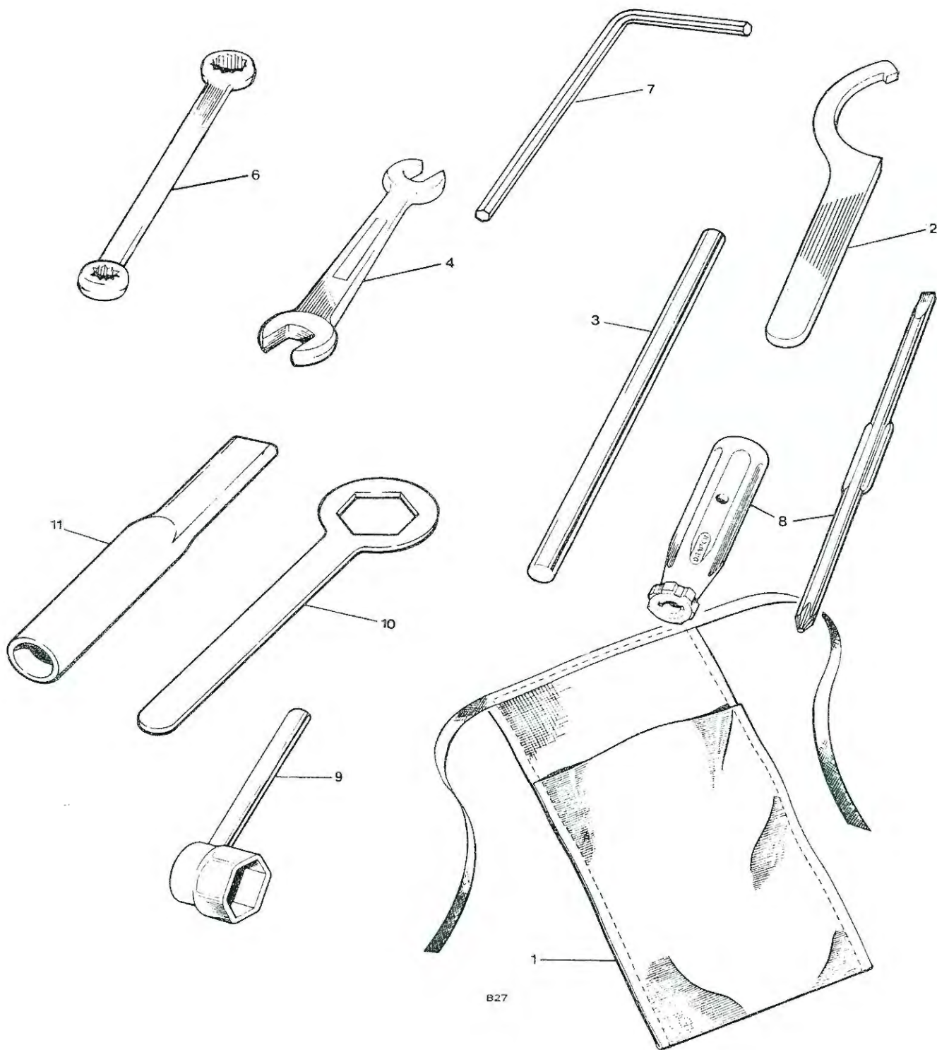
TOOLKIT
