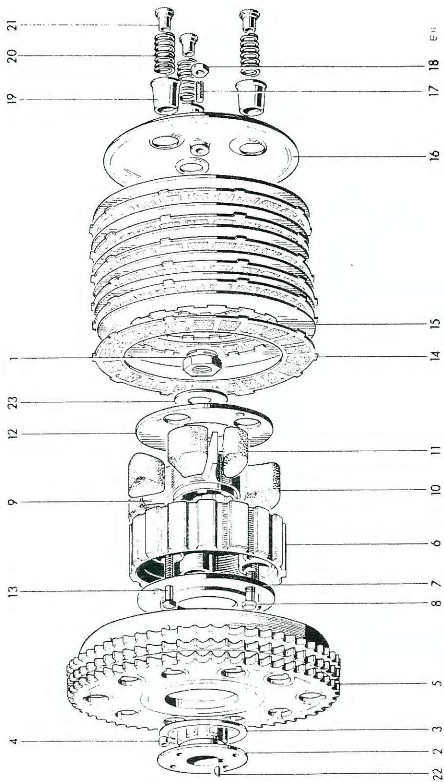
CLUTCH
