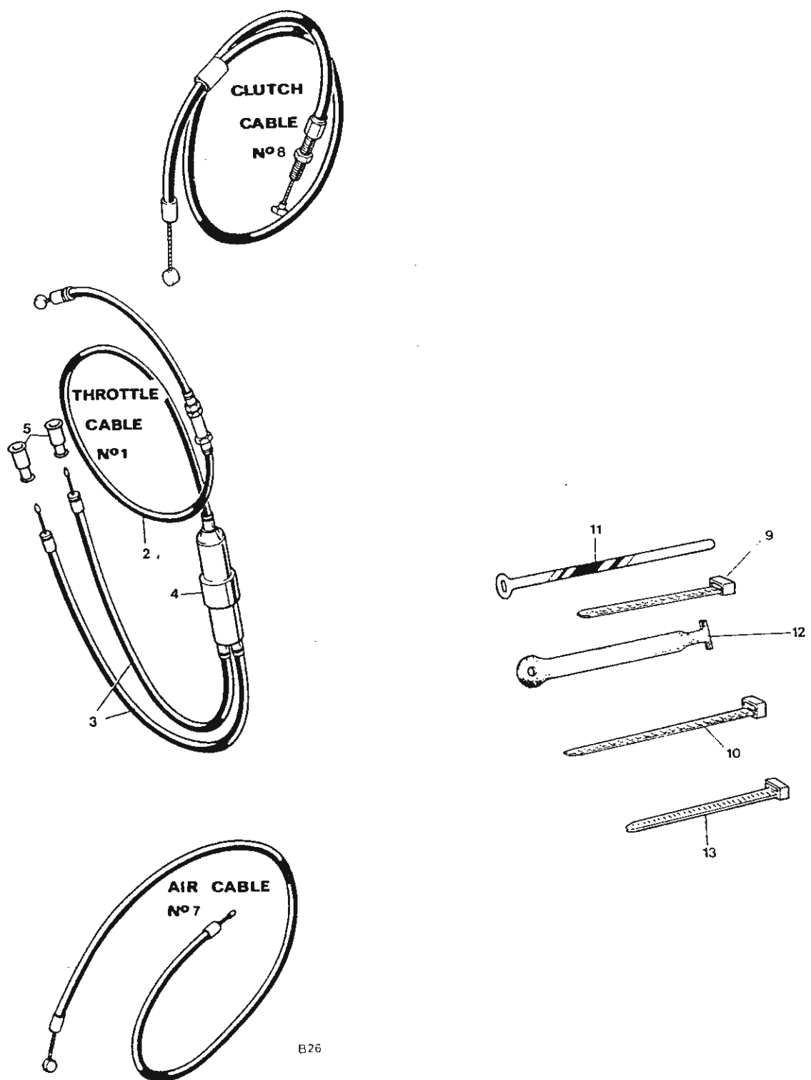
Fig. 30. CONTROL CABLES
