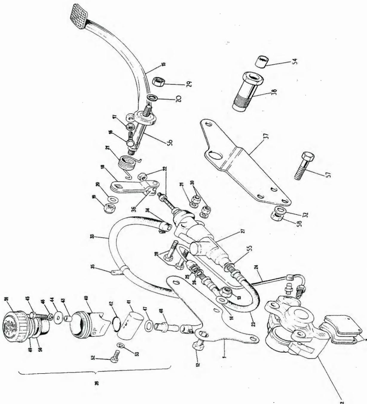
FIG. 25. REAR BRAKE
