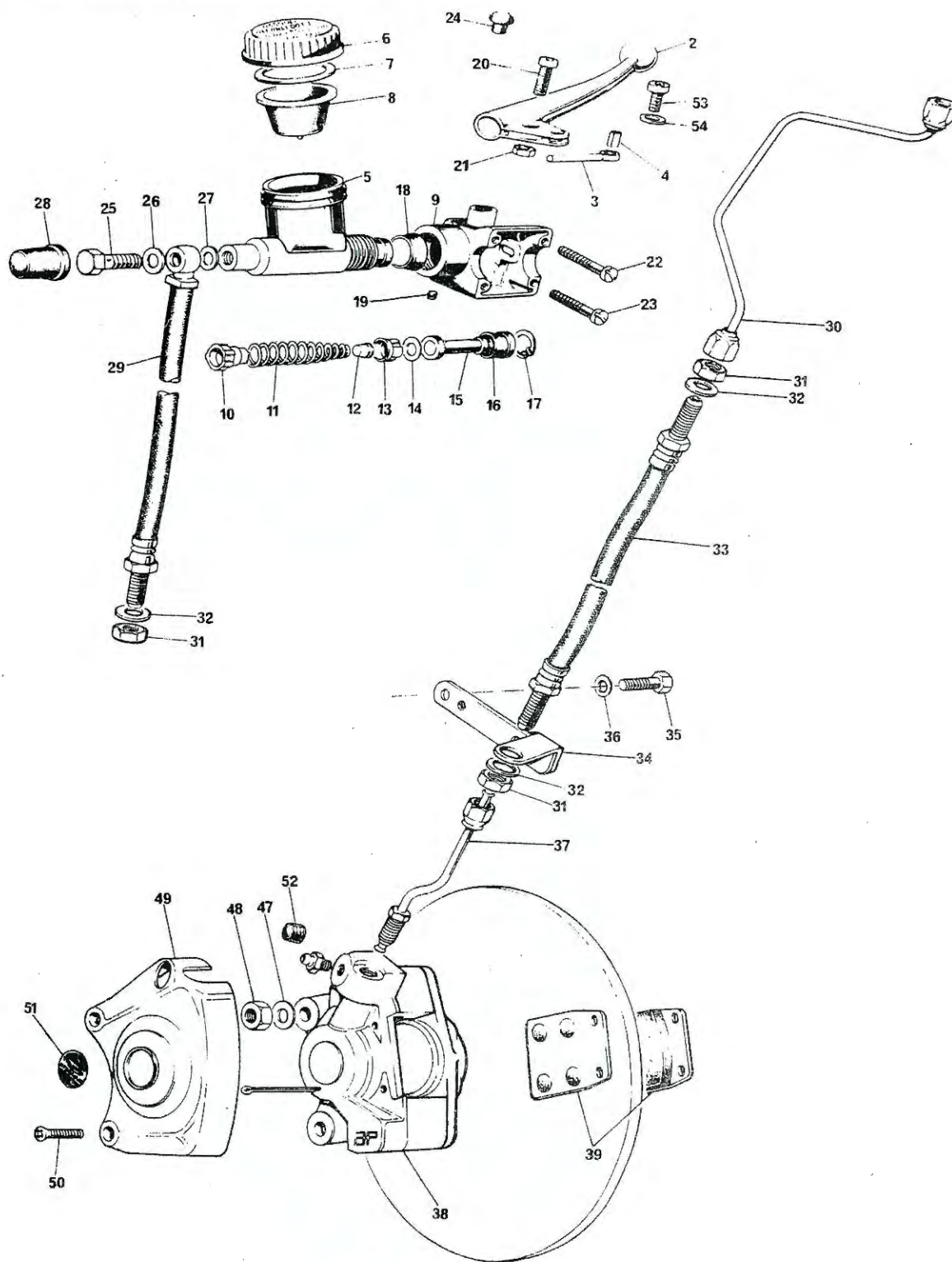
Fig. 23. FRONT BRAKE
