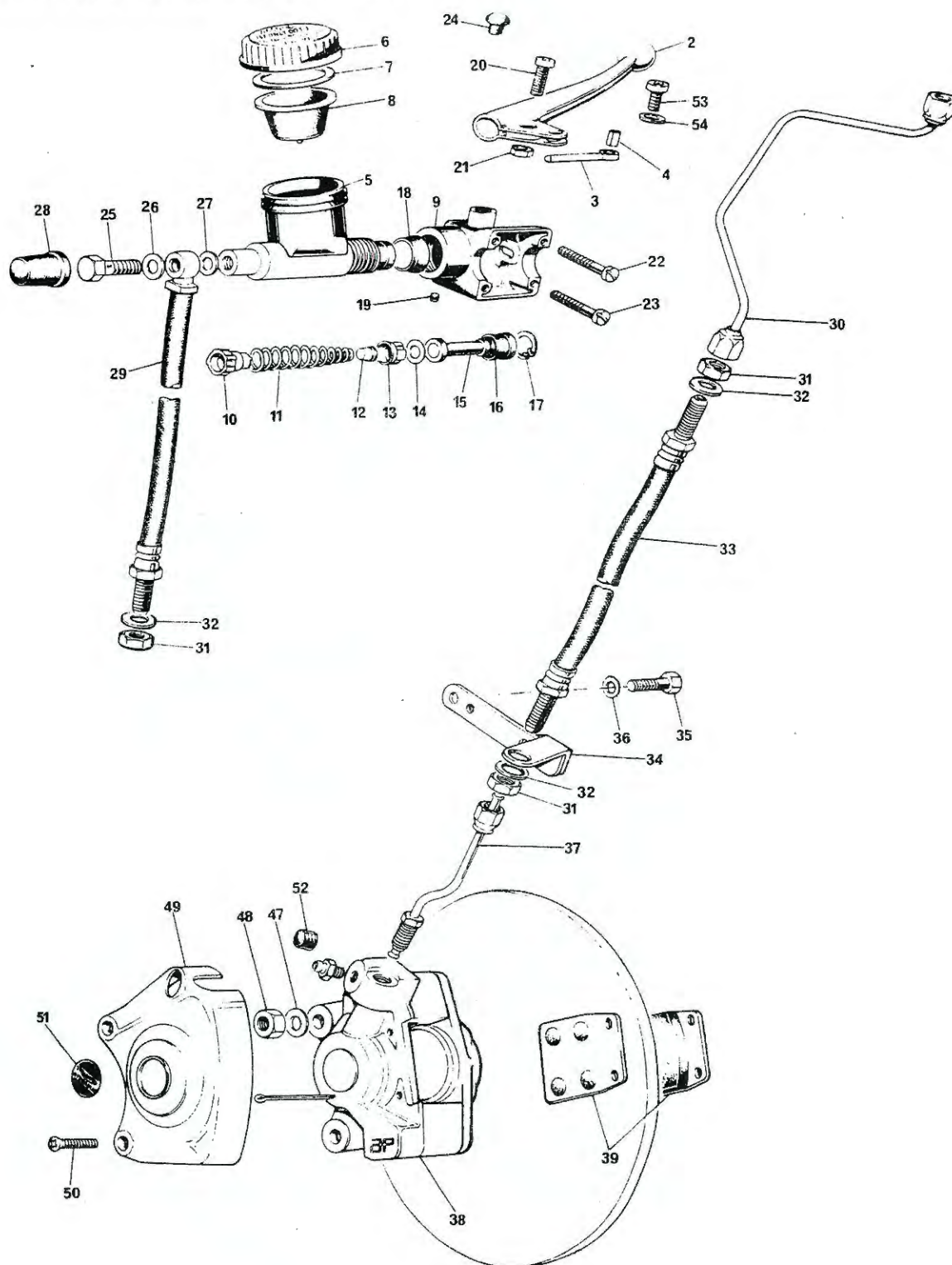
Fig. 23. FRONT BRAKE
