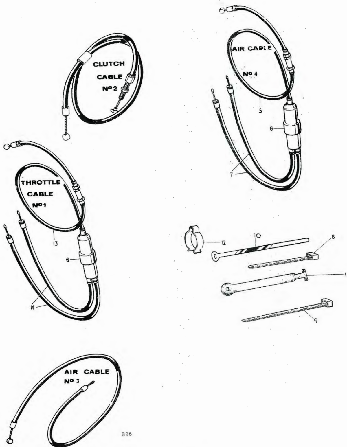
Fig. 30. CONTROL CABLES
