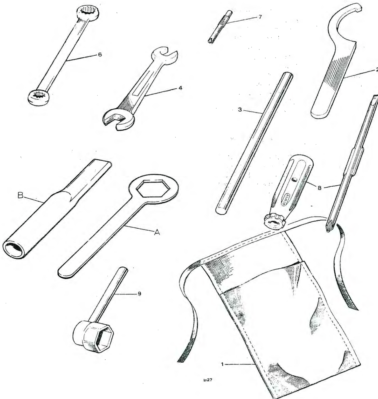
Fig. 31. TOOLKIT
