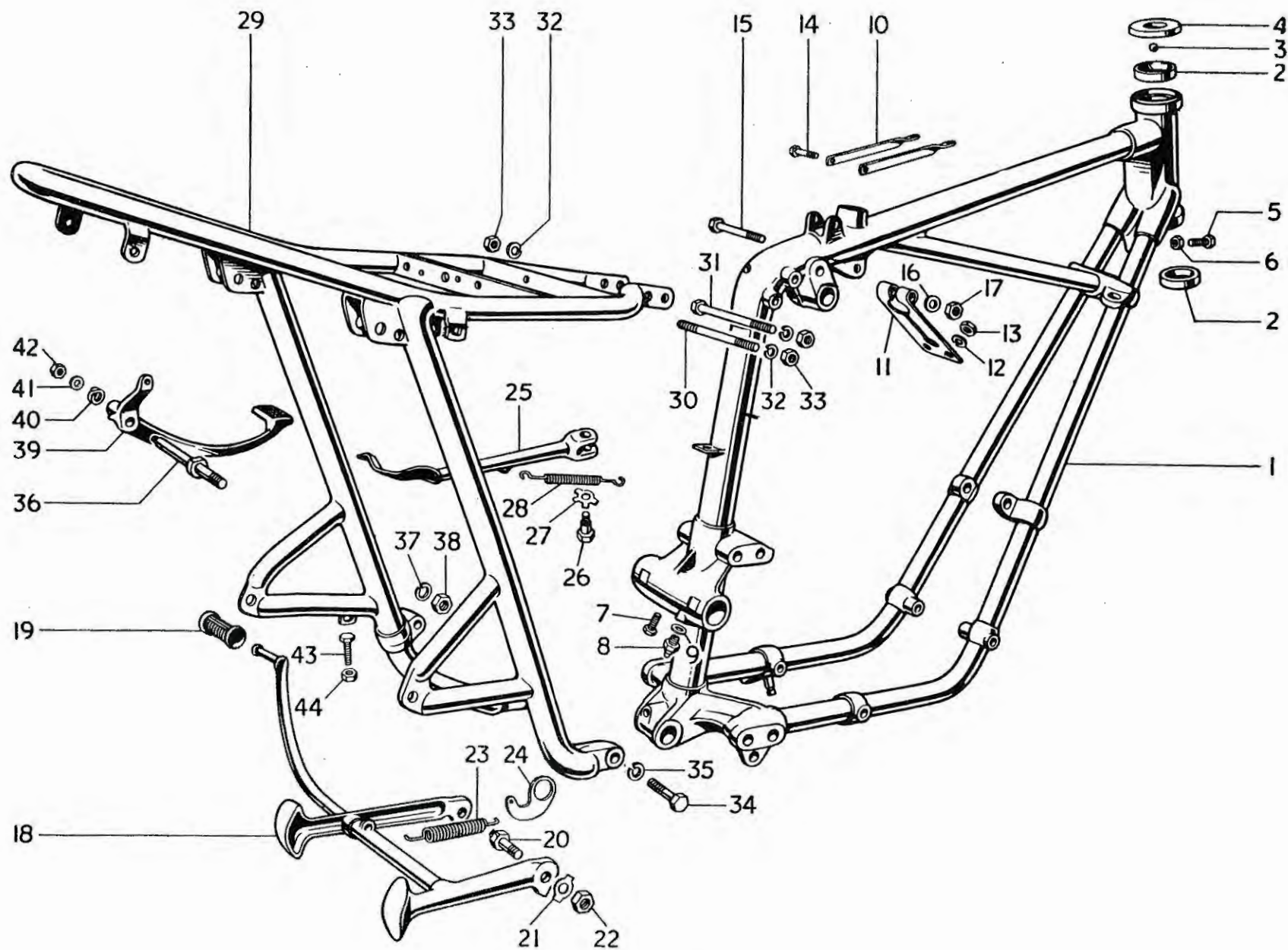
FIG. 11 FRAME
