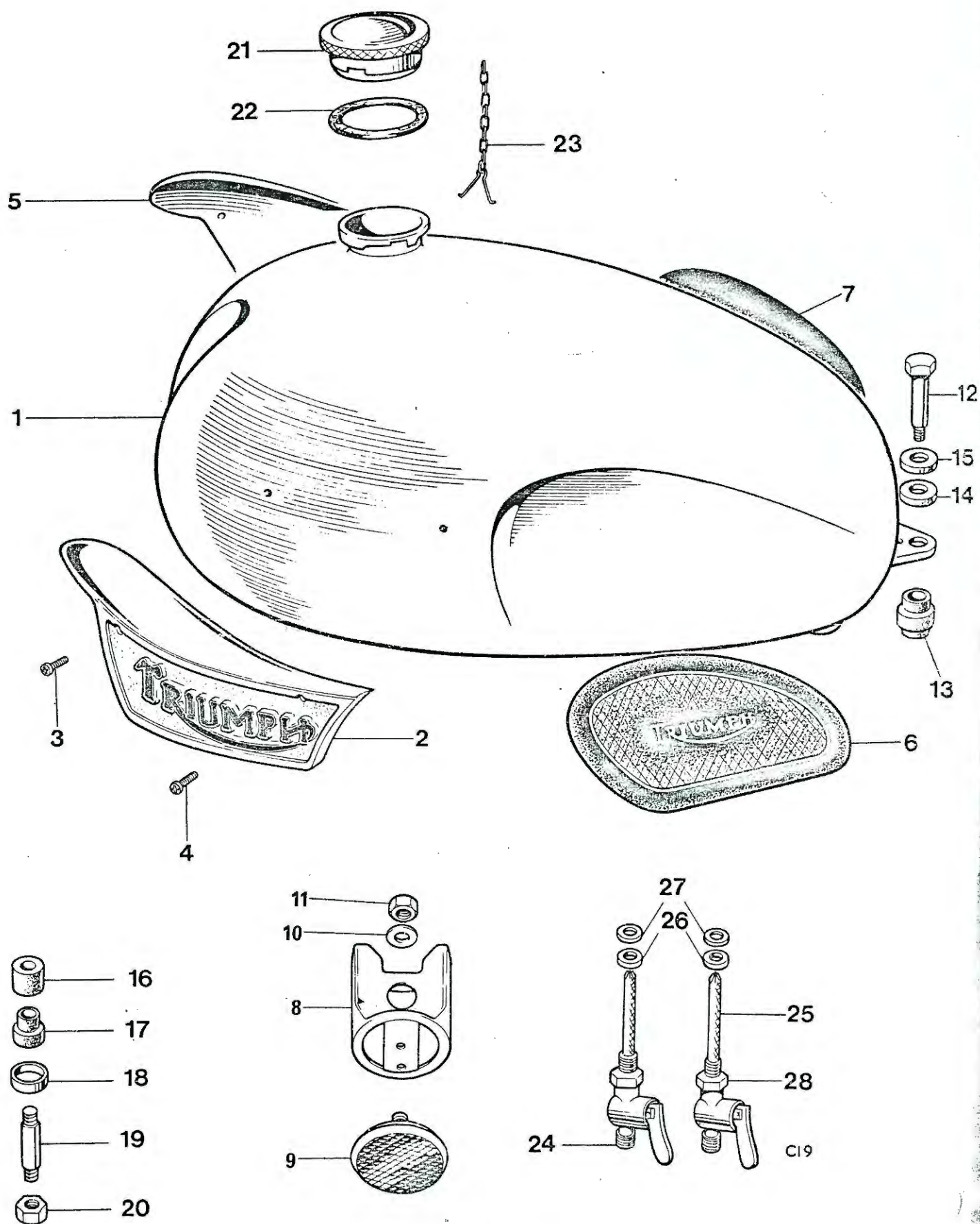
Fig. 22. GAS TANK
