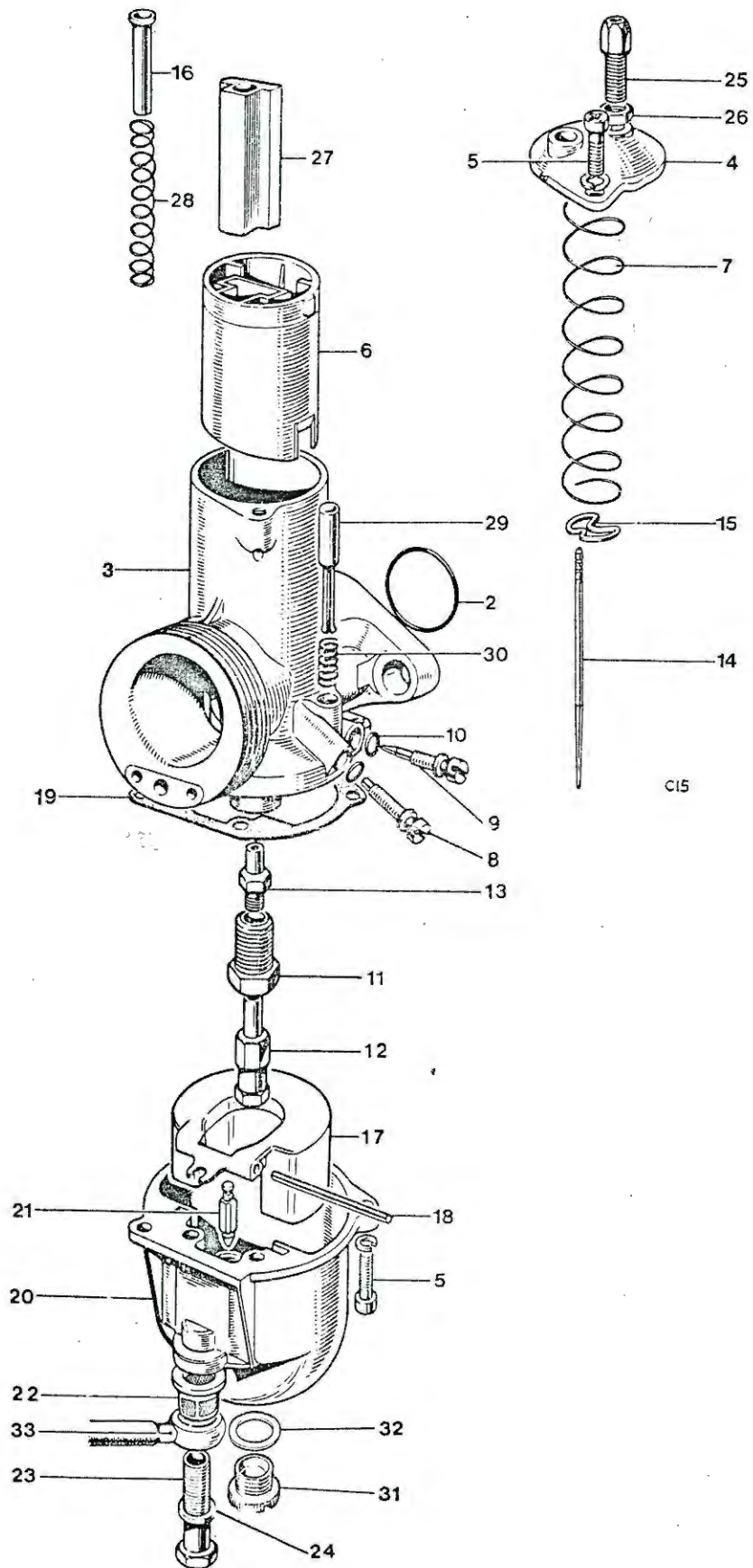
Fig. 5. CARBURETOR
