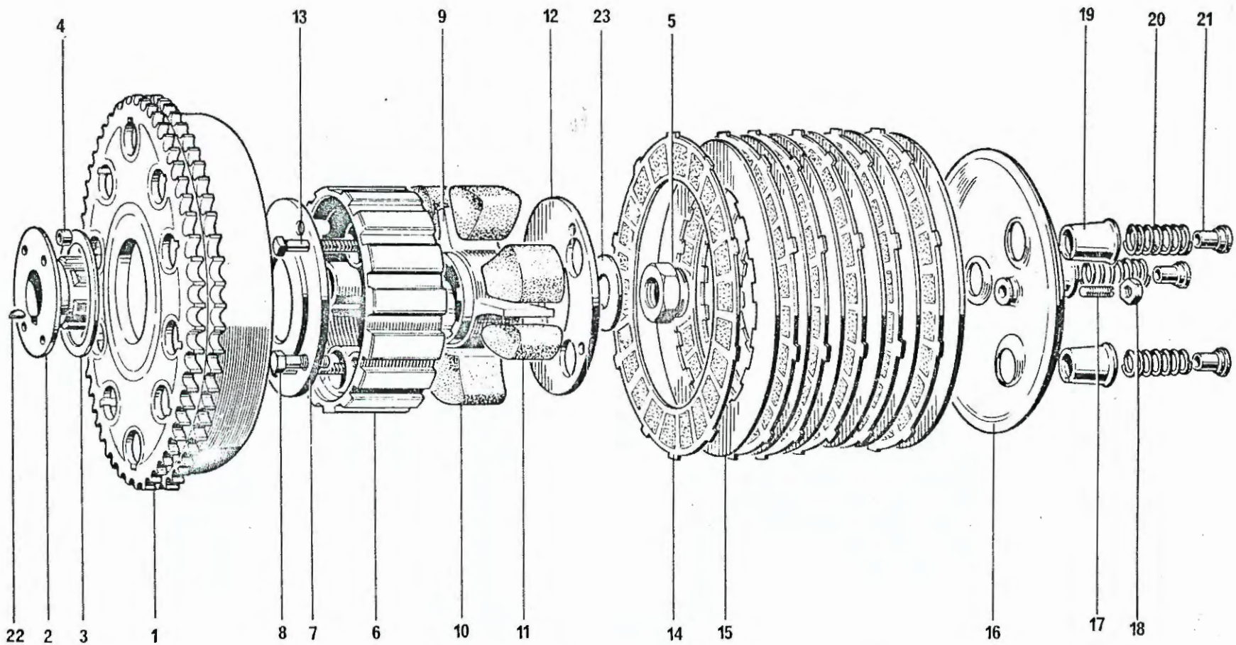
Fig. 10. CLUTCH
