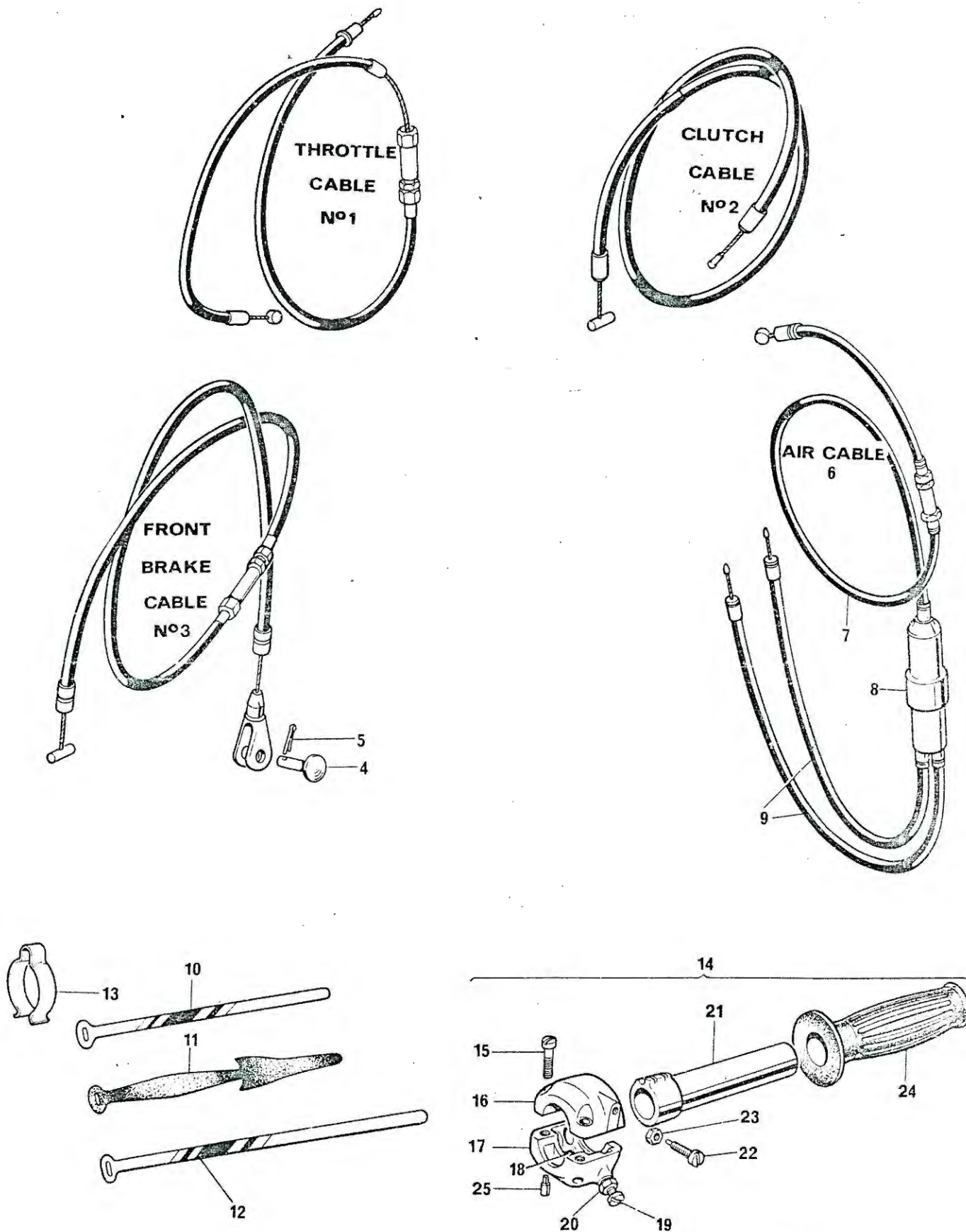
Fig. 26. CONTROL CABLES
