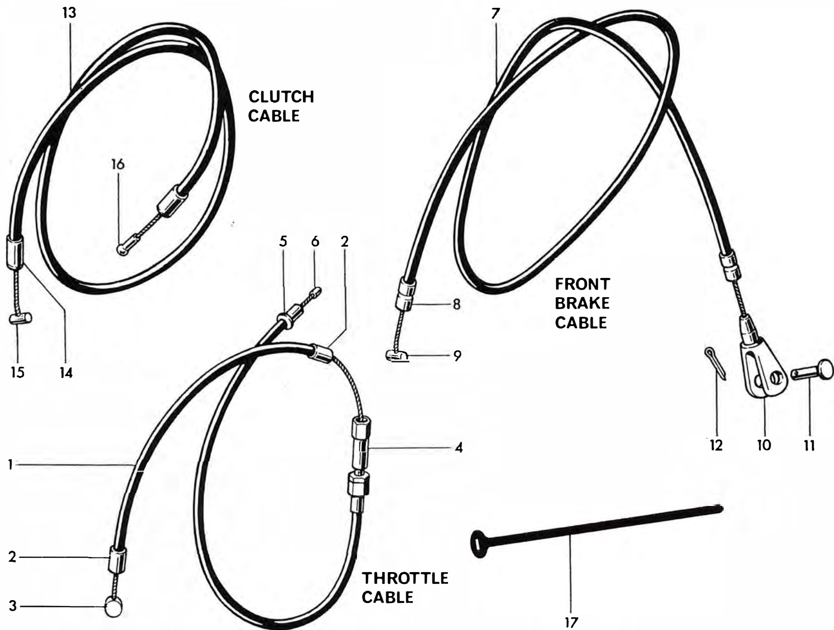
Fig. 29. CONTROL CABLES
