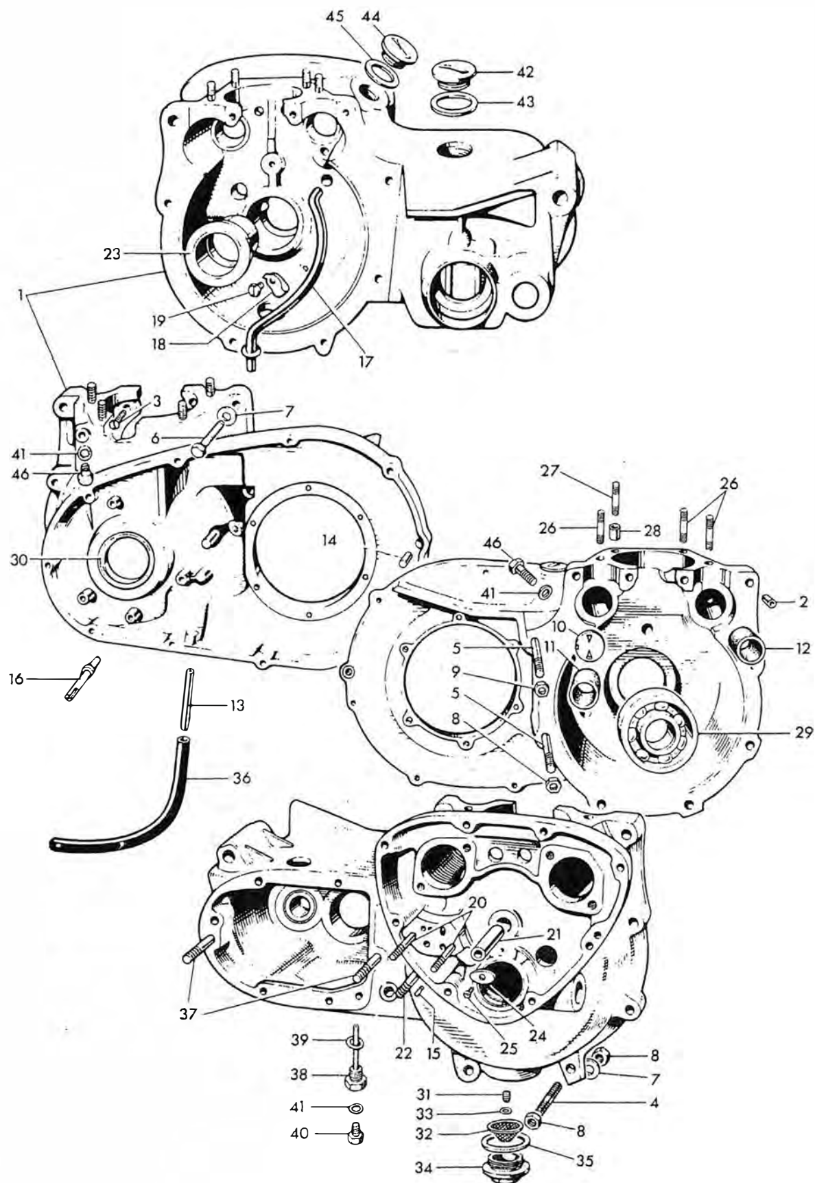
Fig. 2. CRANKCASE
