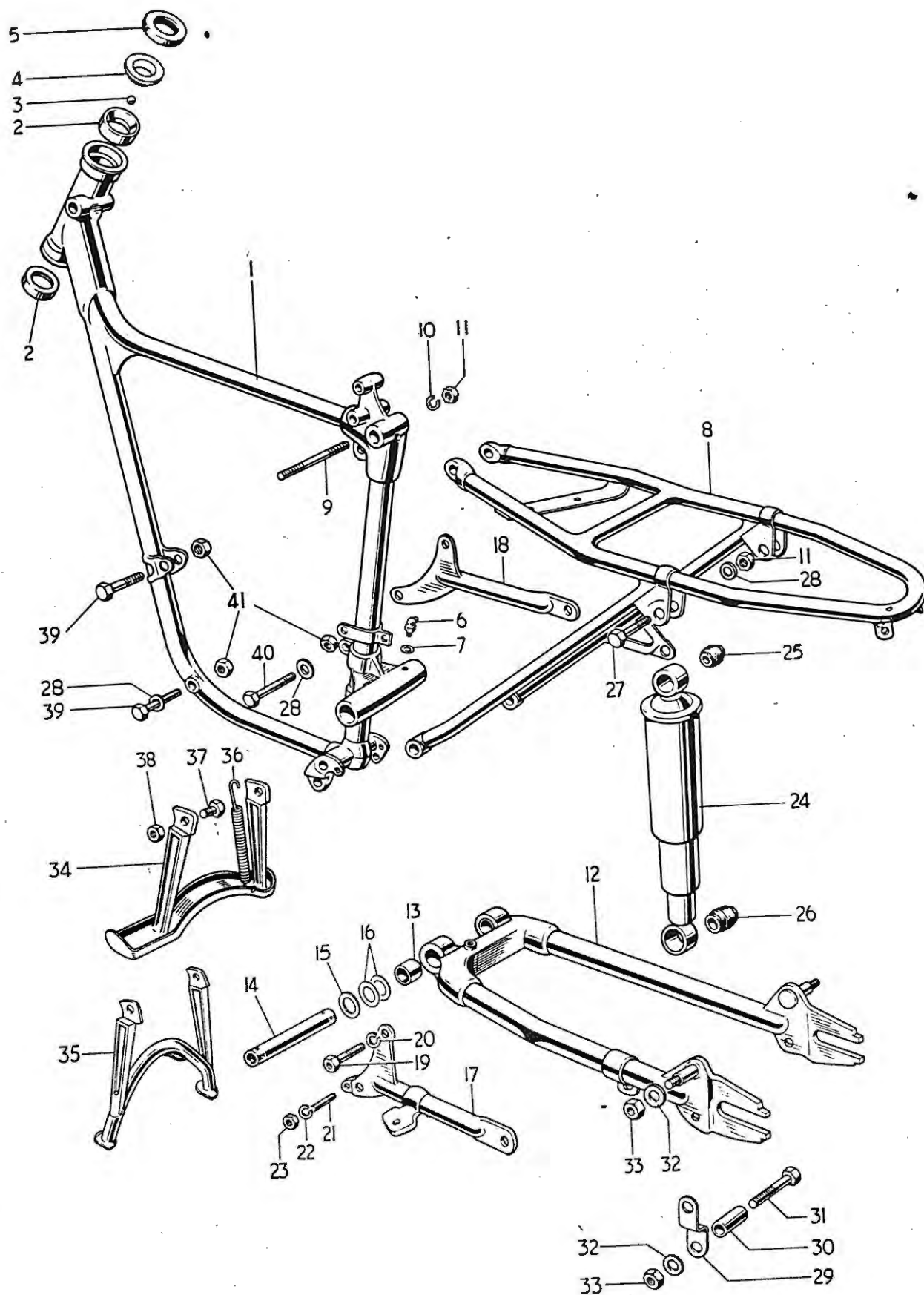
Fig. 7. FRAME COMPLETE
