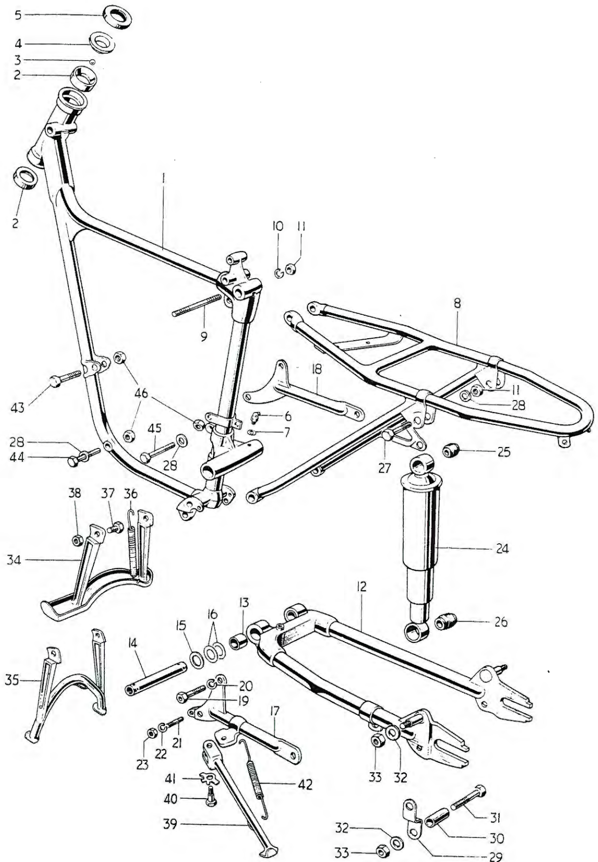
Fig. 9. FRAME COMPLETE
