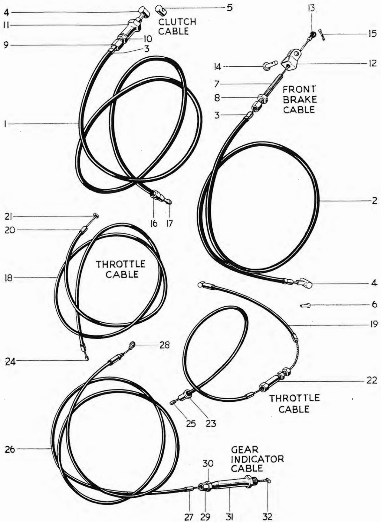
Fig. 23. CONTROL CABLES.
