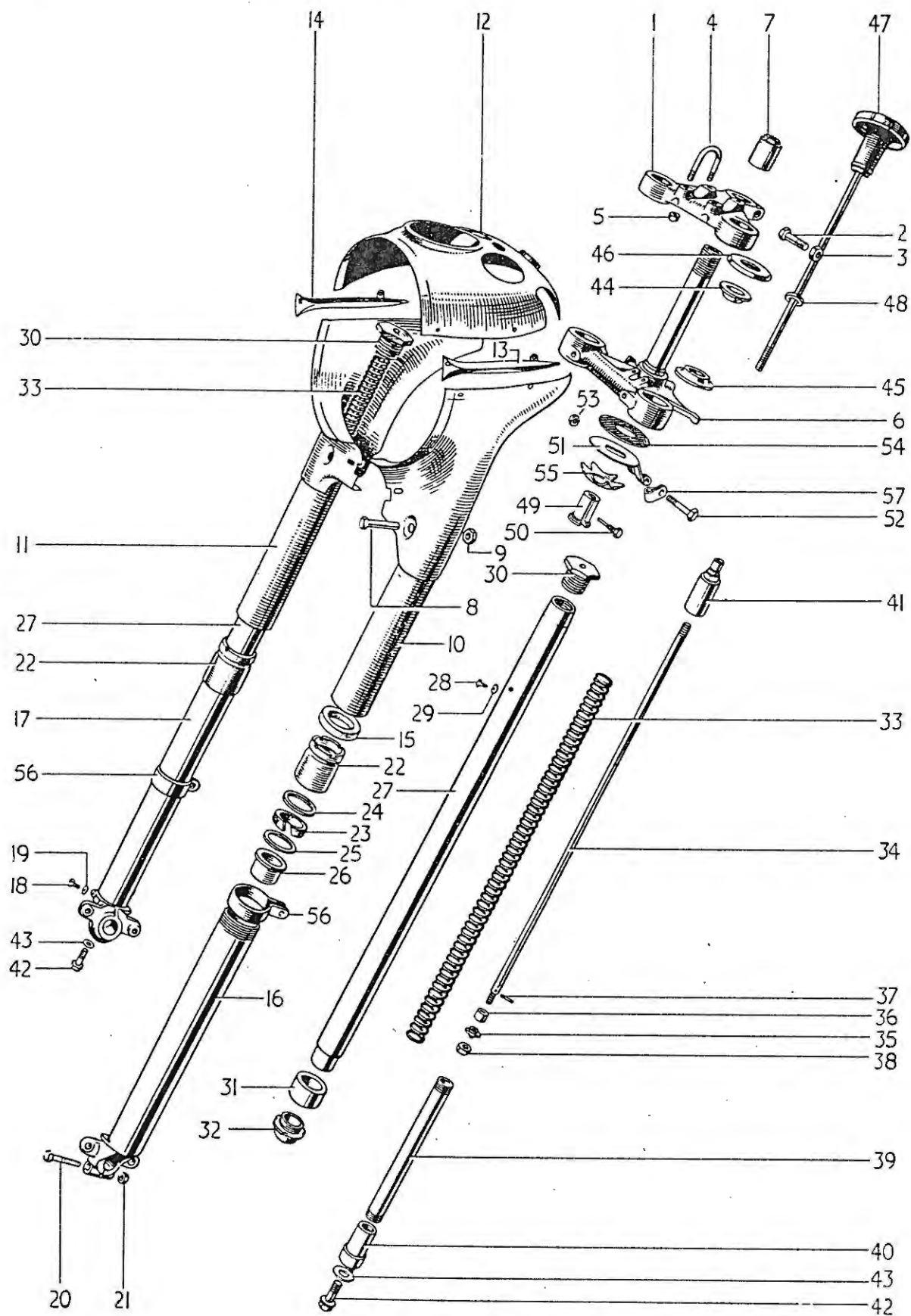
FIG. 16. TELESCOPIC FORK
