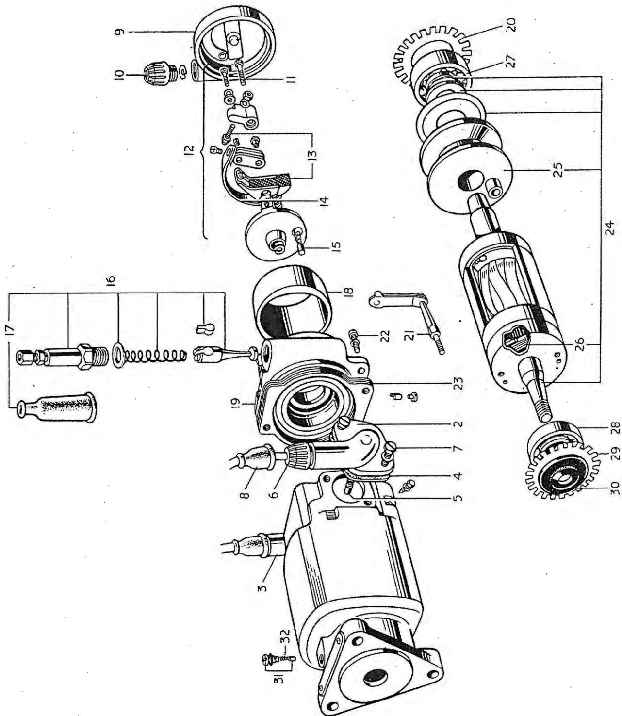
FIG. 33. LUCAS MAGNETO
