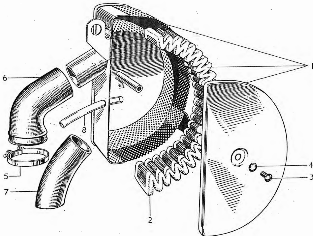
FIG. 29. AIR FILTER
