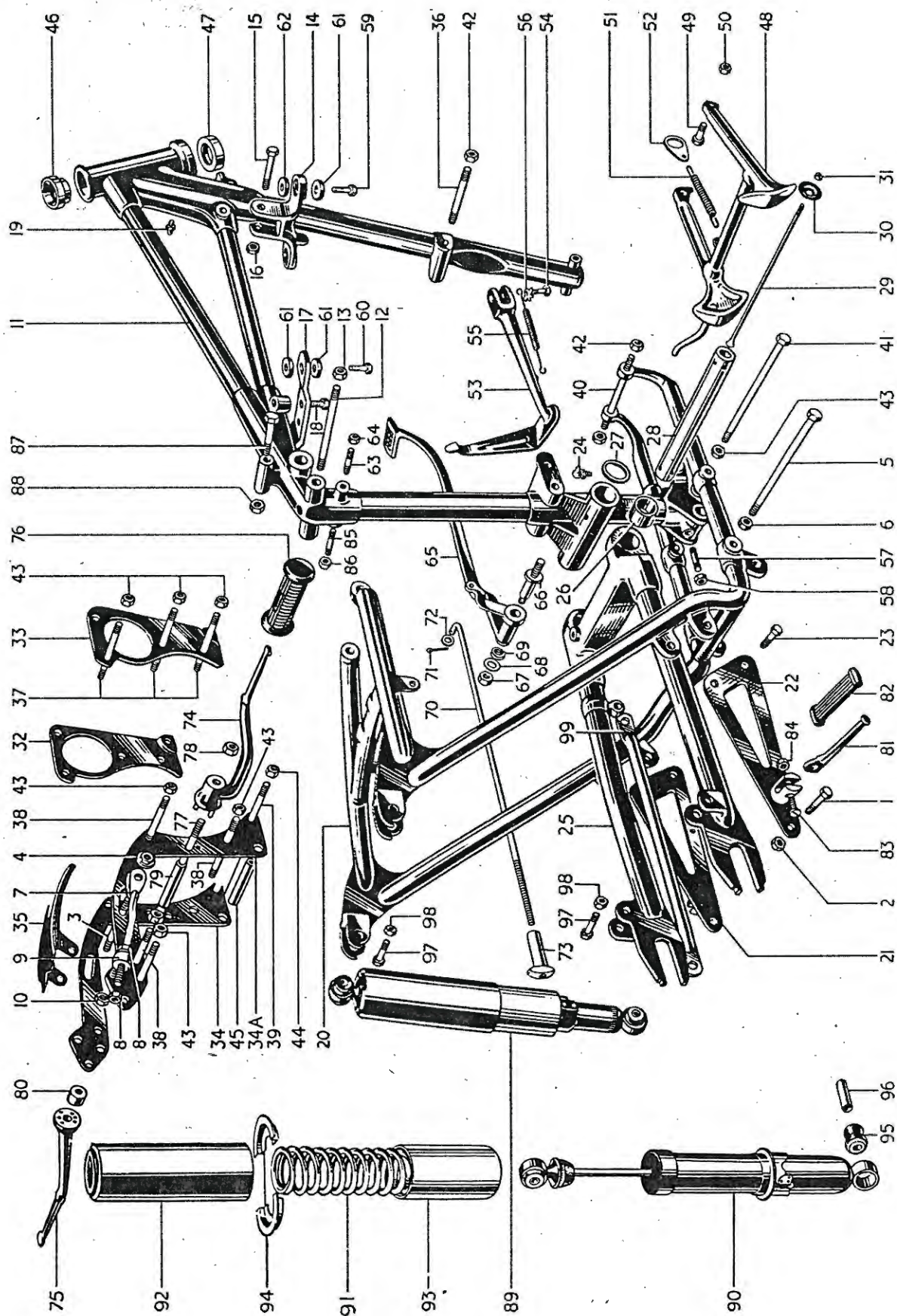
FIG. 13. FRAME
