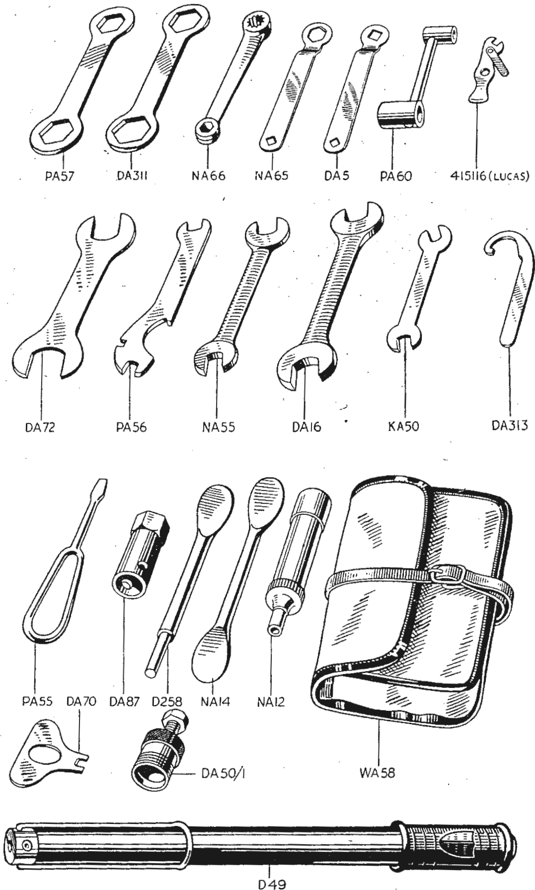
FIG. 28. TOOL KIT
