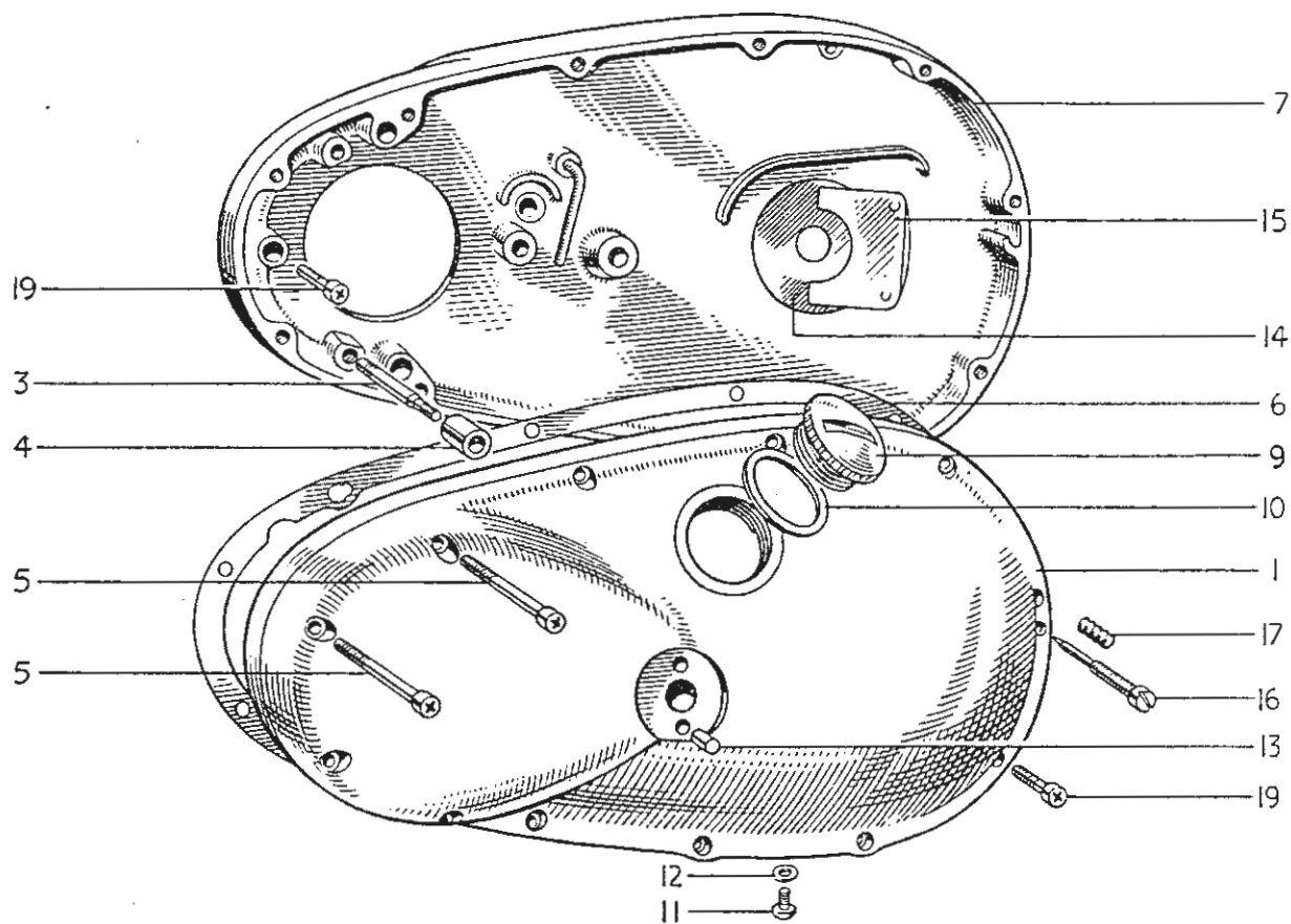
FIG. 25. PRIMARY CHAINCASE
