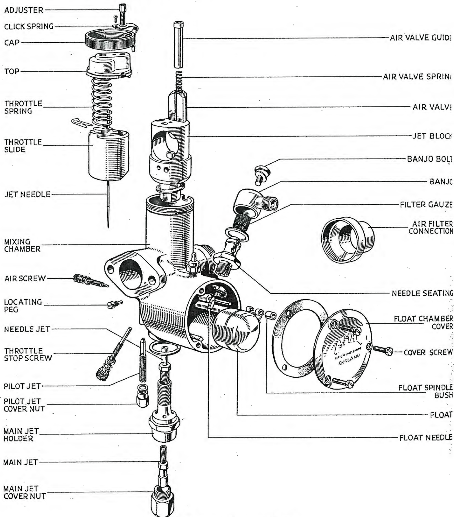
FIG. 30. AMAL CARBURETTER
