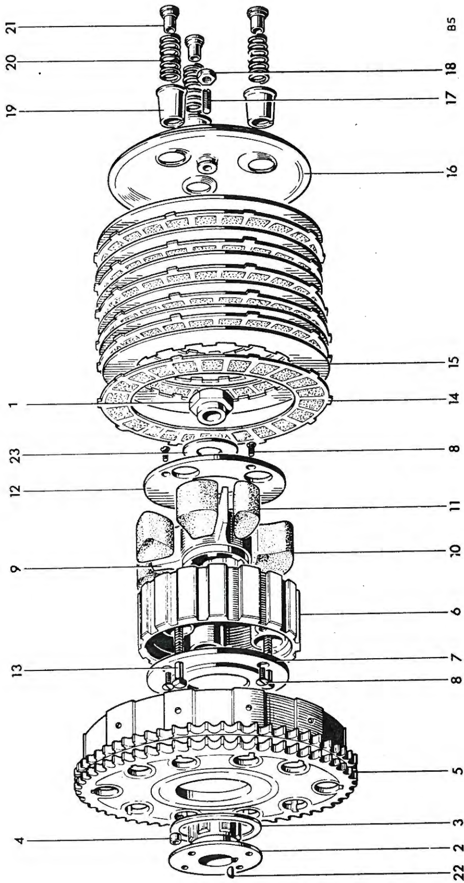
Fig. 10. CLUTCH
