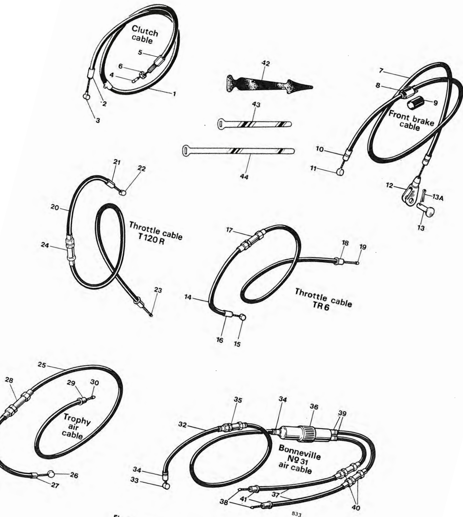
Fig. 27. CONTROL CABLES
