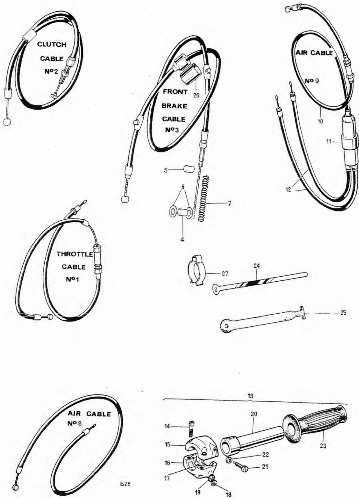
Fig. 30. CONTROL CABLES
