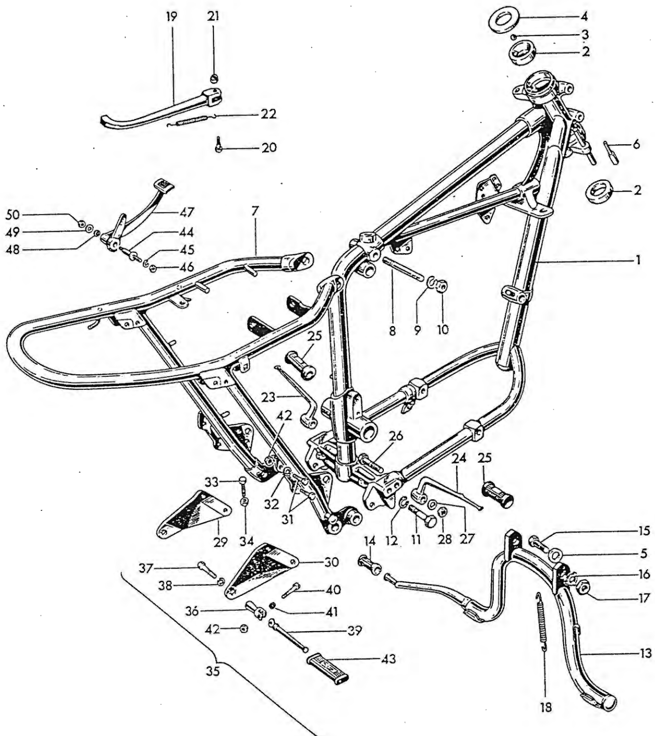
Fig. 15. FRAME
