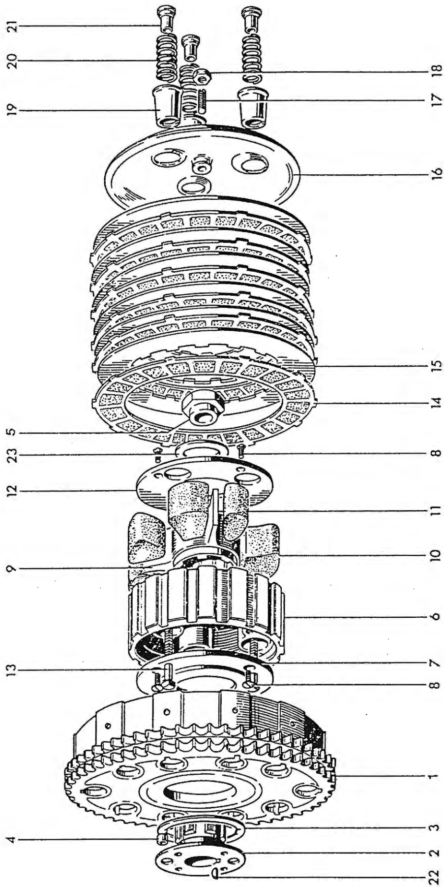
Fig. 11. CLUTCH
