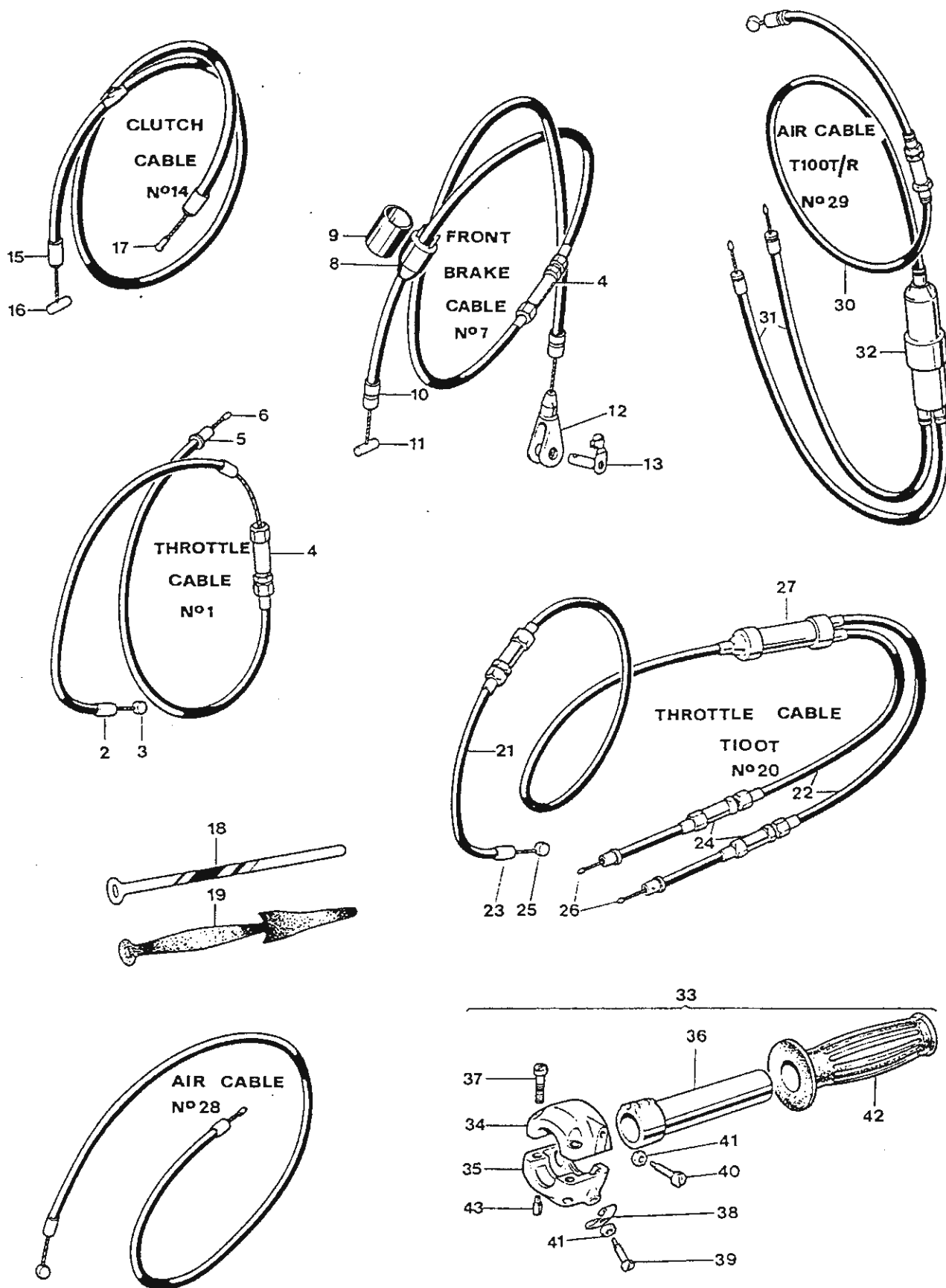
Fig. 29. CONTROL CABLES
