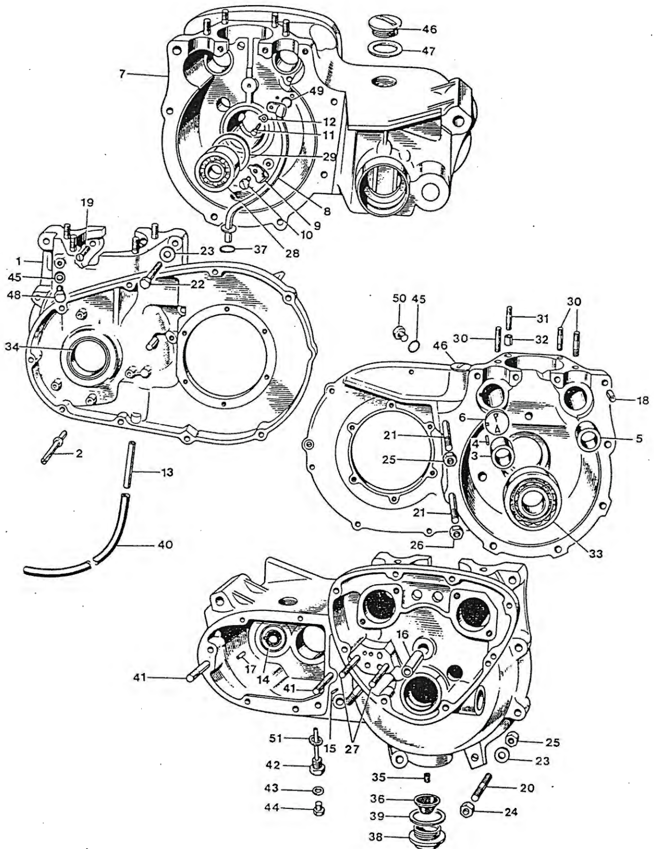
Fig. 2. CRANKCASE
