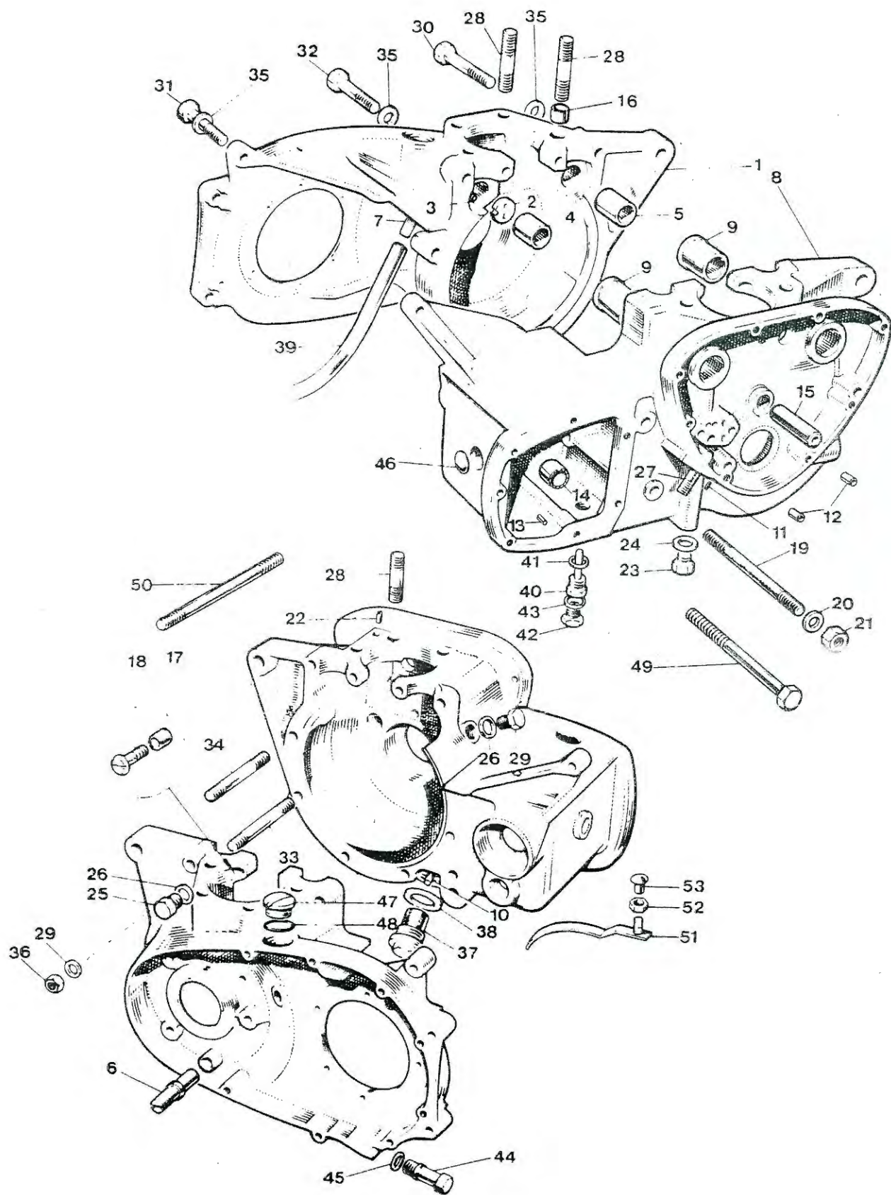
Fig. 2. CRANKCASE
