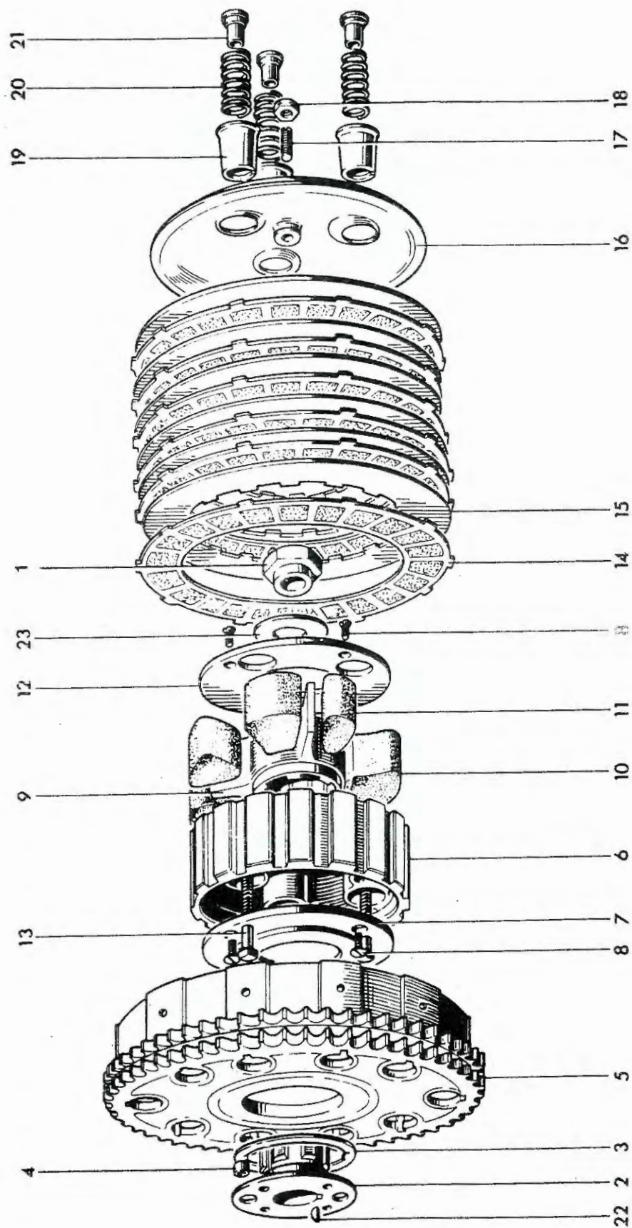
Fig. 10. CLUTCH
