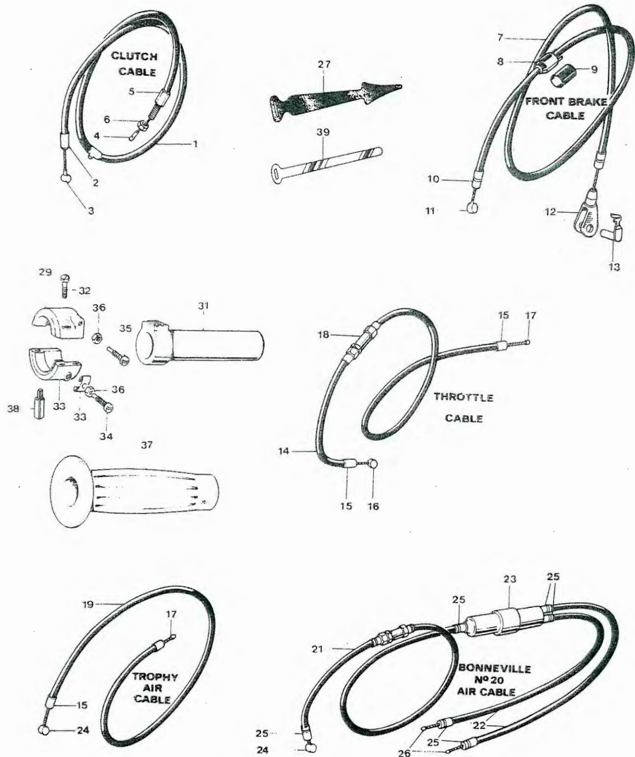
Fig. 28. CONTROL CABLES
