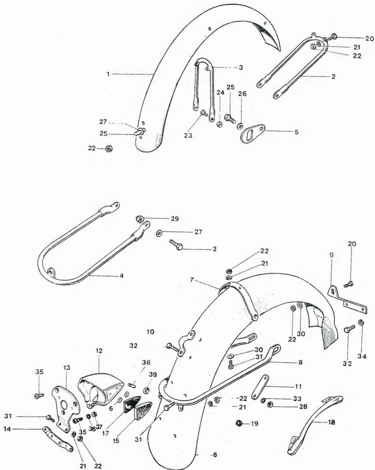
Fig. 26. FENDERS
