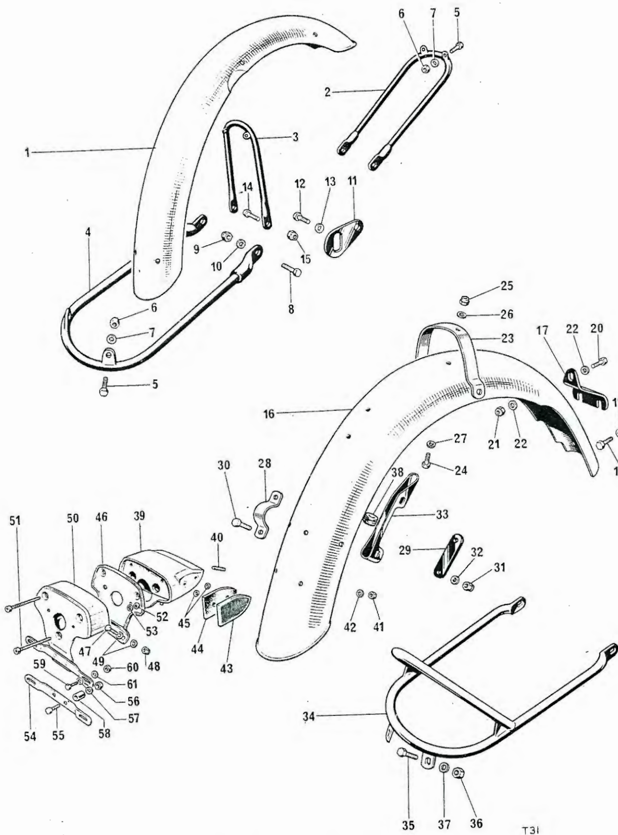
Fig. 28. MUDGUARDS (FENDERS)
