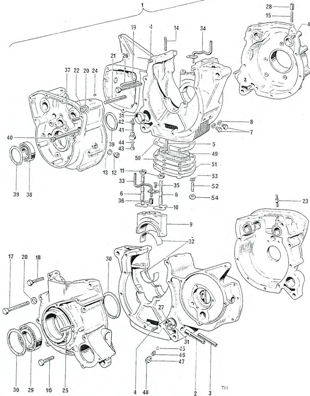
Fig. 2. CRANKCASES
