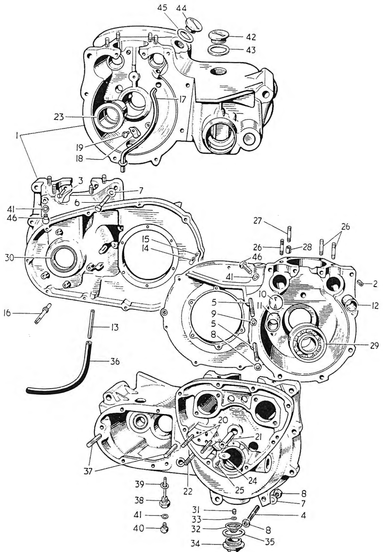
Fig. 2. CRANKCASE
