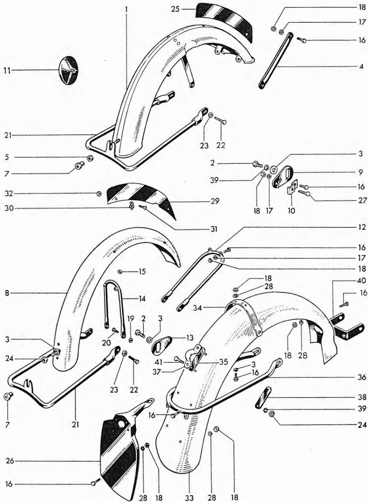
Fig. 20. MUDGUARDS
