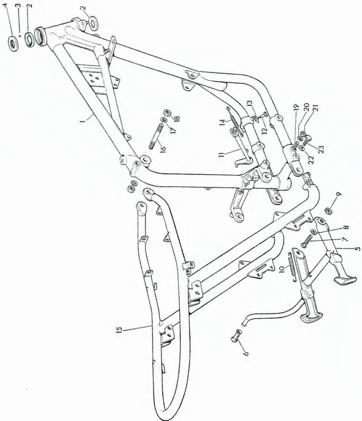
Fig. 12. FRAME
