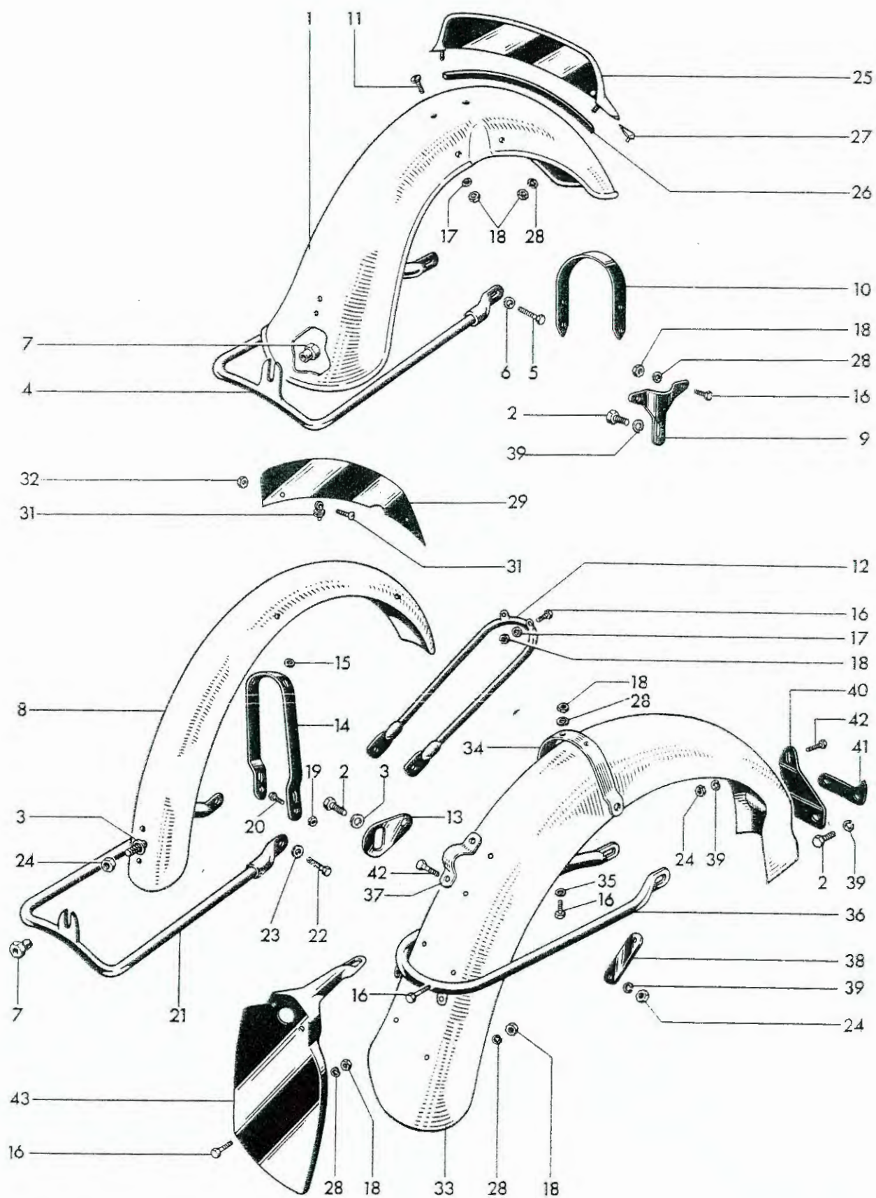
Fig. 26. MUDGUARDS
