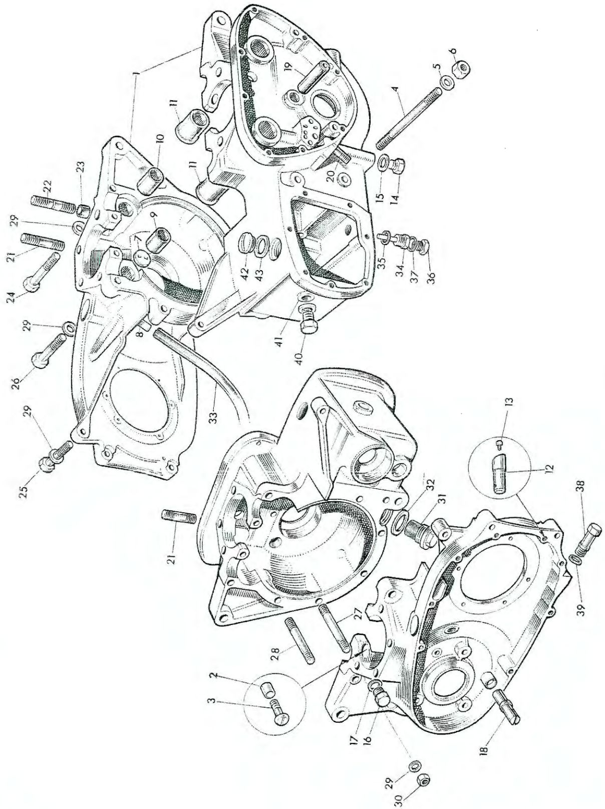
Fig. 2. CRANKCASE
