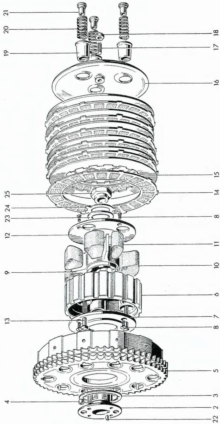
Fig. 10. CLUTCH
