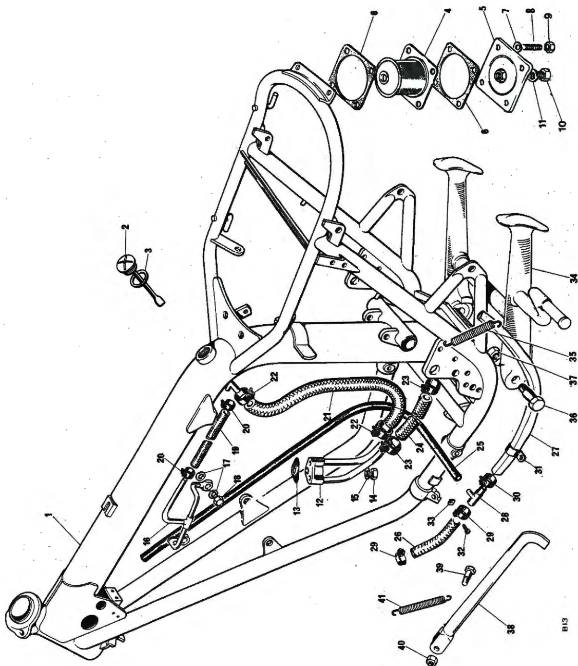
16. FRAME
