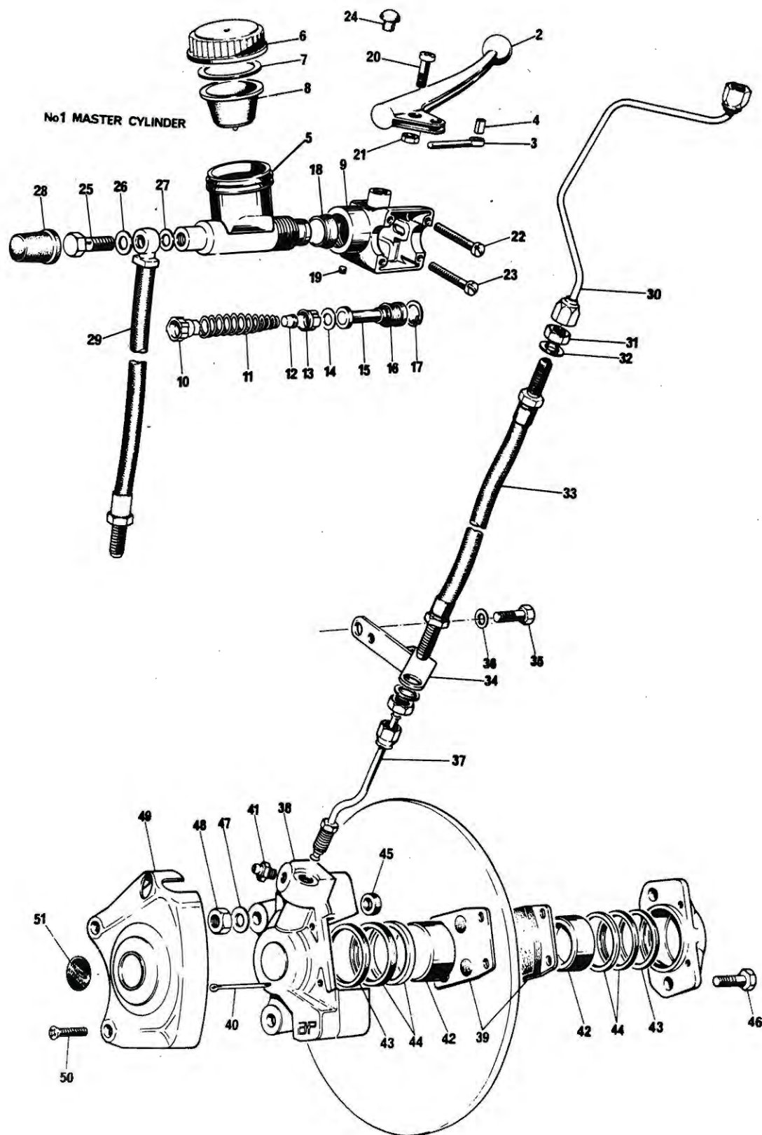
Fig. 23. FRONT BRAKE
