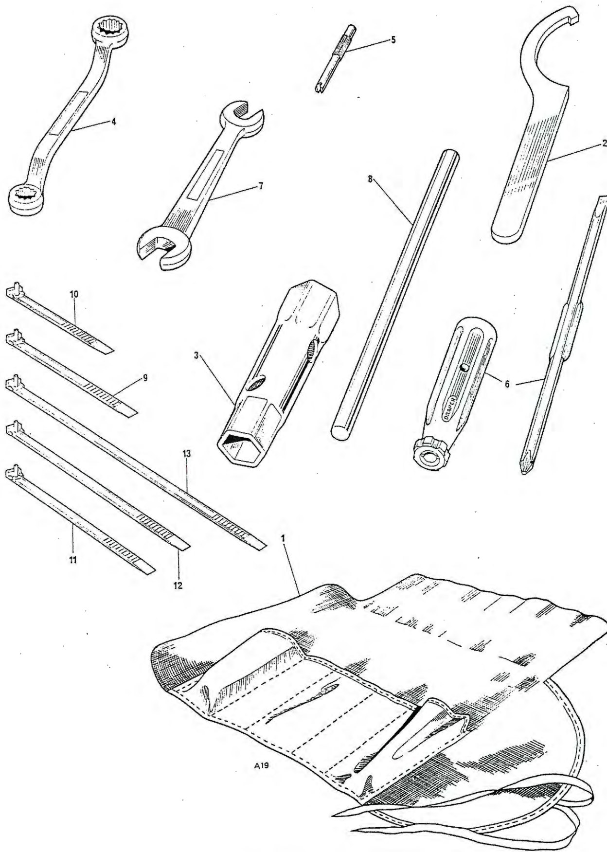
Fig. 19. TOOL KIT
