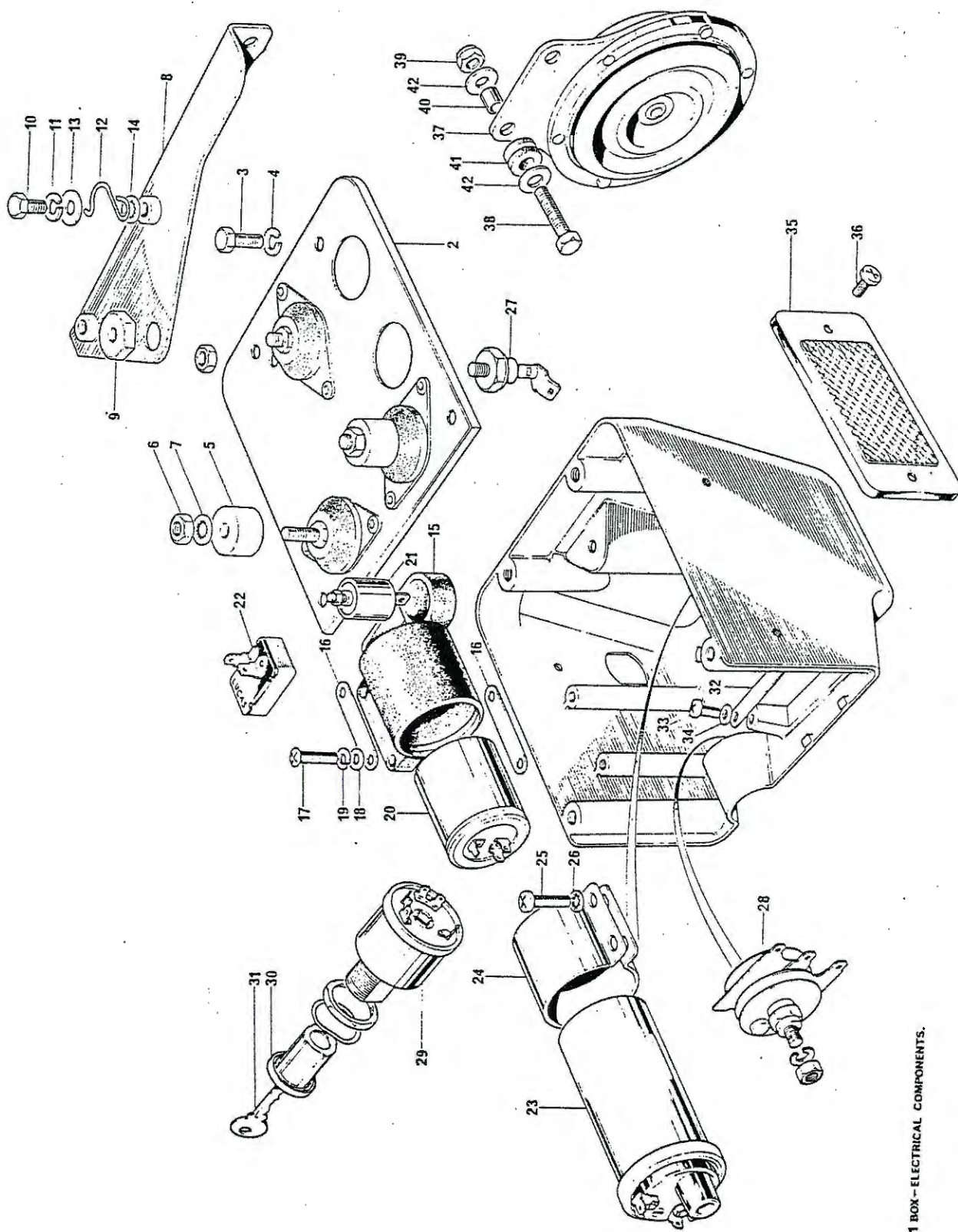
Fig. 17. ELECTRICAL BOX
