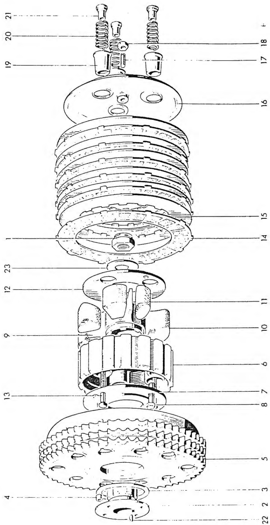
CLUTCH
