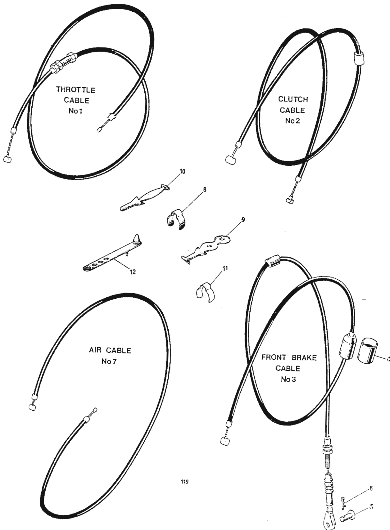
Fig. 21. CONTROL CABLES
