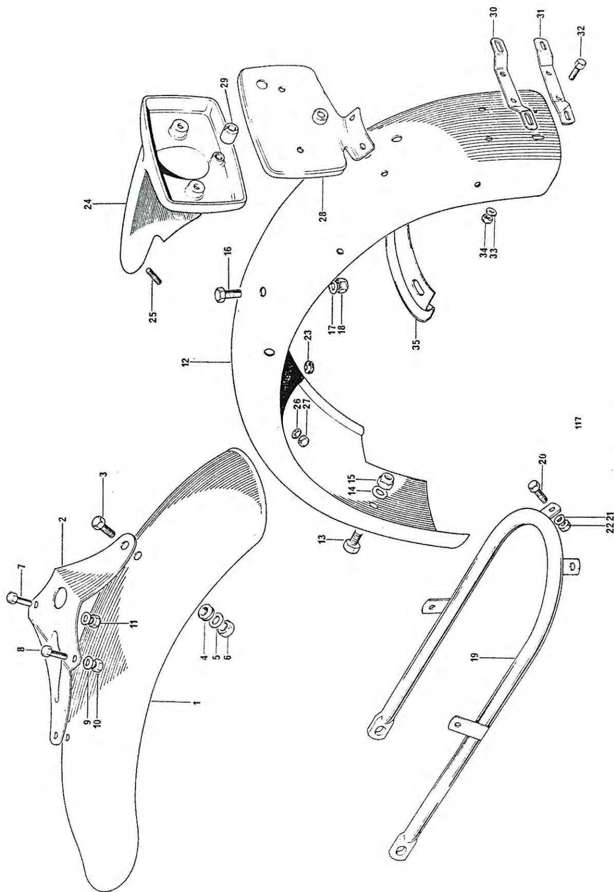
Fig. 19. FENDERS
