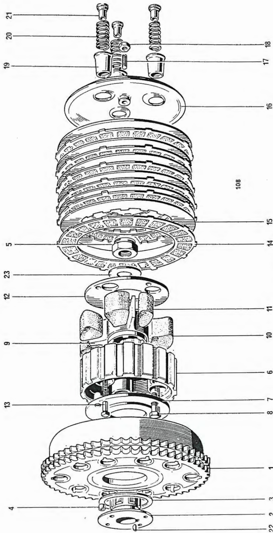
Fig. 10. CLUTCH
