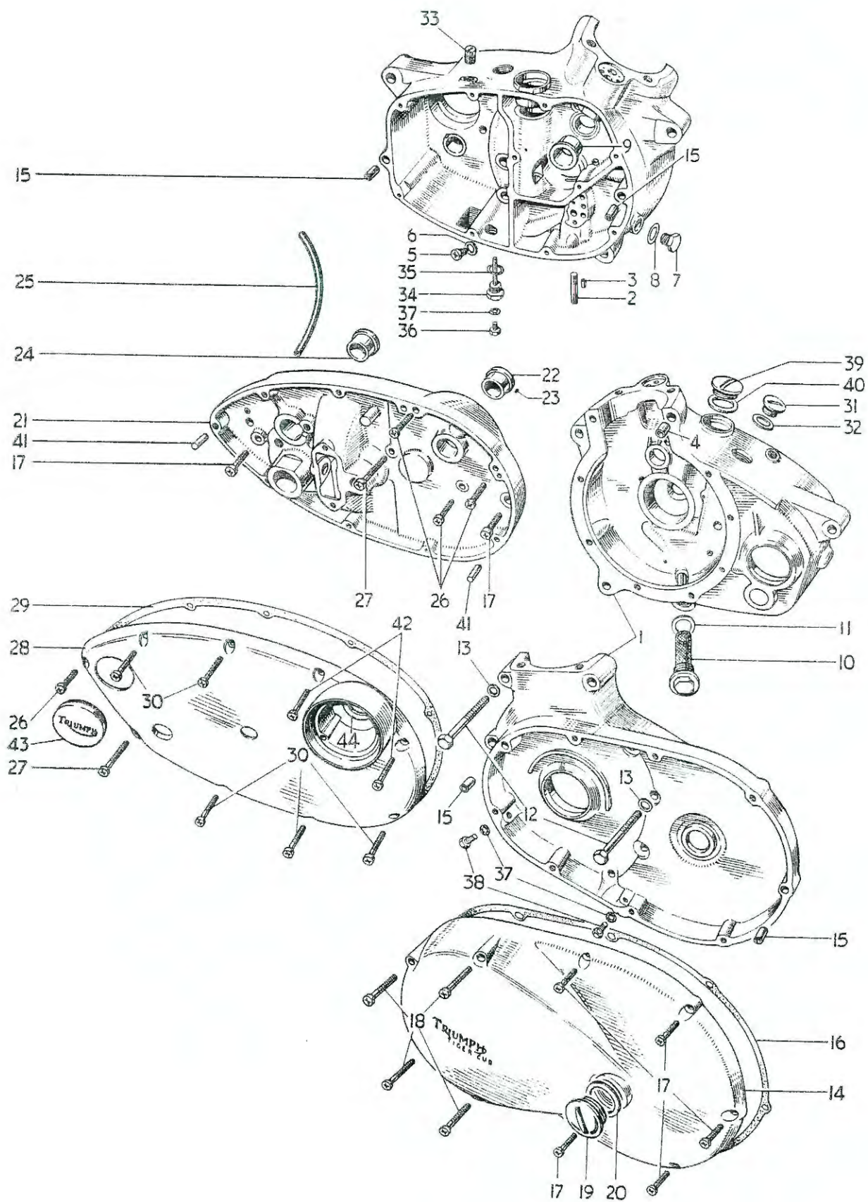
Fig. 2. CRANKCASE
