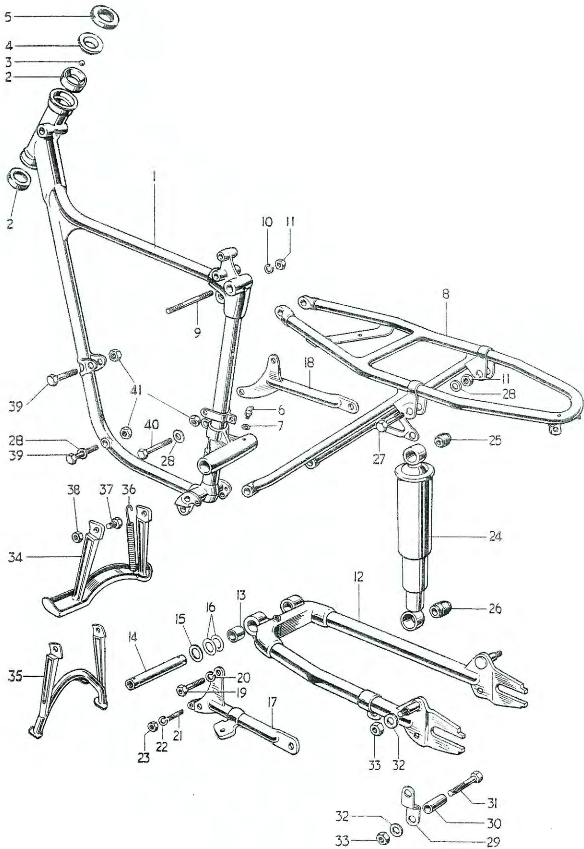
Fig. 7. FRAME COMPLETE
