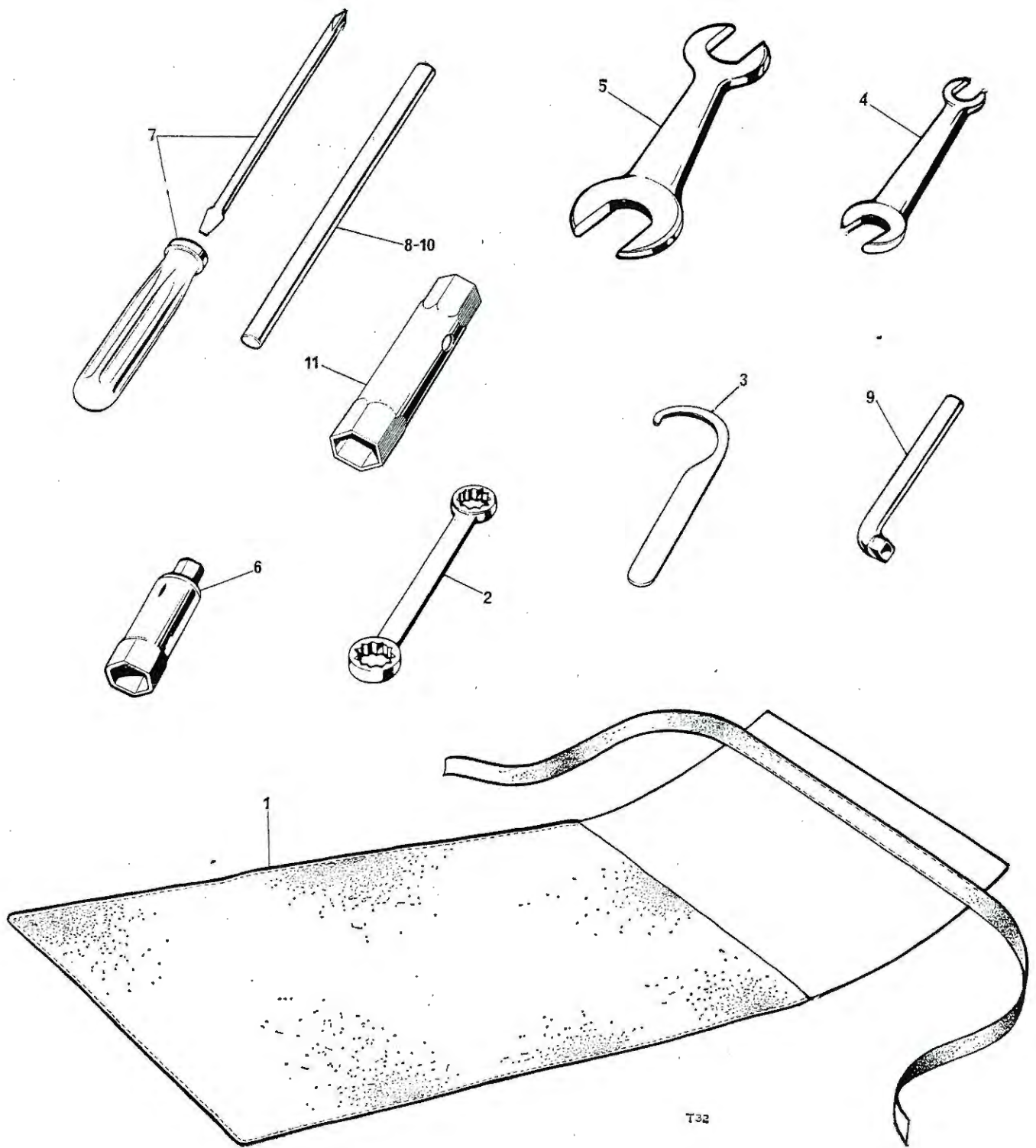
Fig. 32. TOOLKIT
