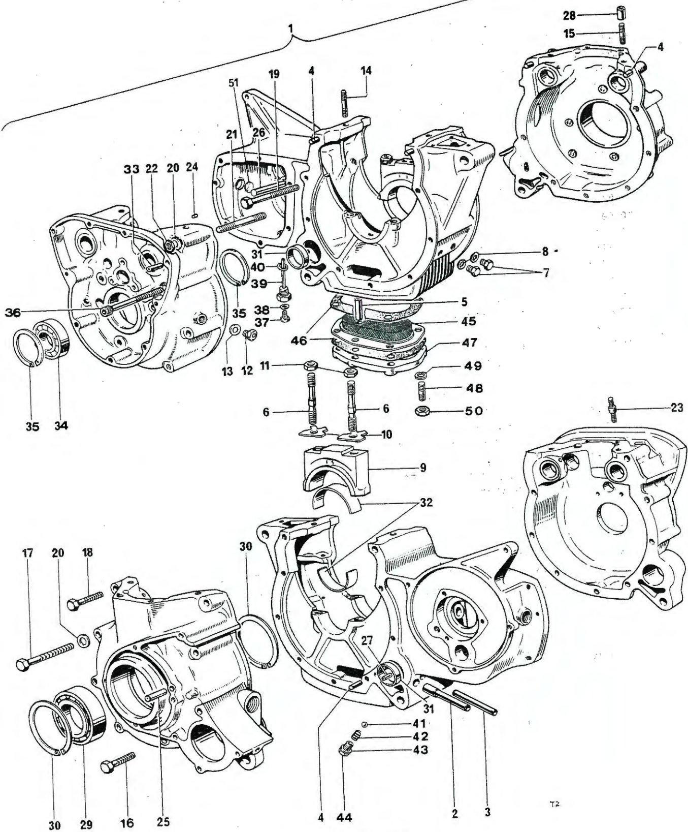
Fig. 2. CRANKCASES
