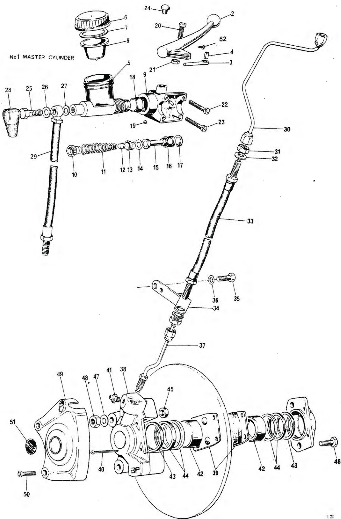
Fig. 21. FRONT BRAKE
