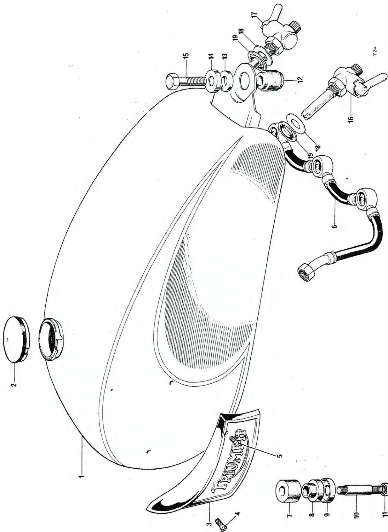
Fig. 24. GAS TANK
