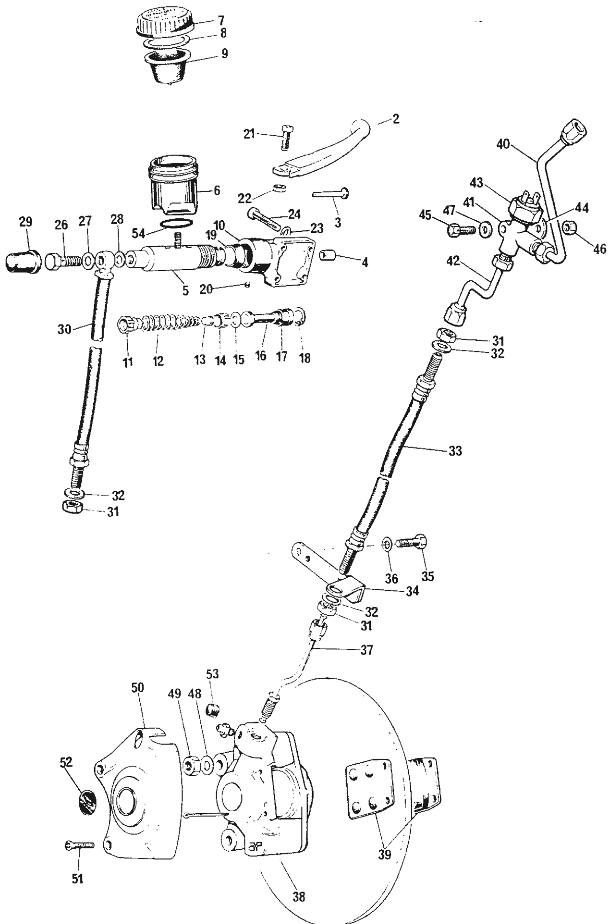
Fig. 23. FRONT BRAKE
