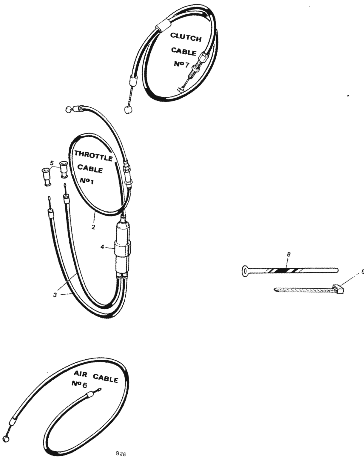
Fig. 30. CONTROL CABLES
