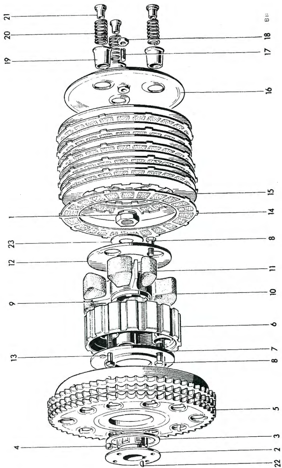
Fig. 14. CLUTCH
