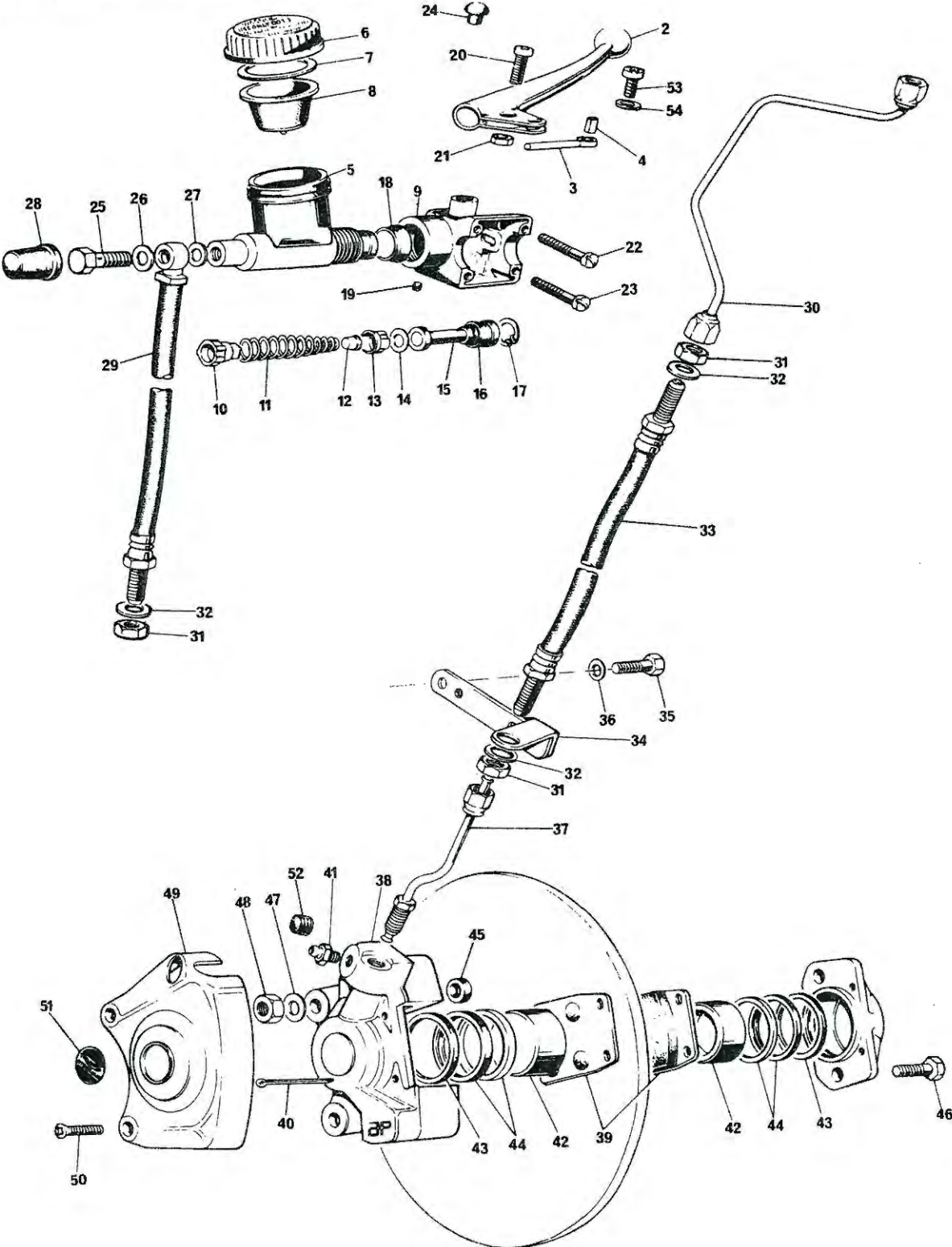
Fig. 23. FRONT BRAKE
