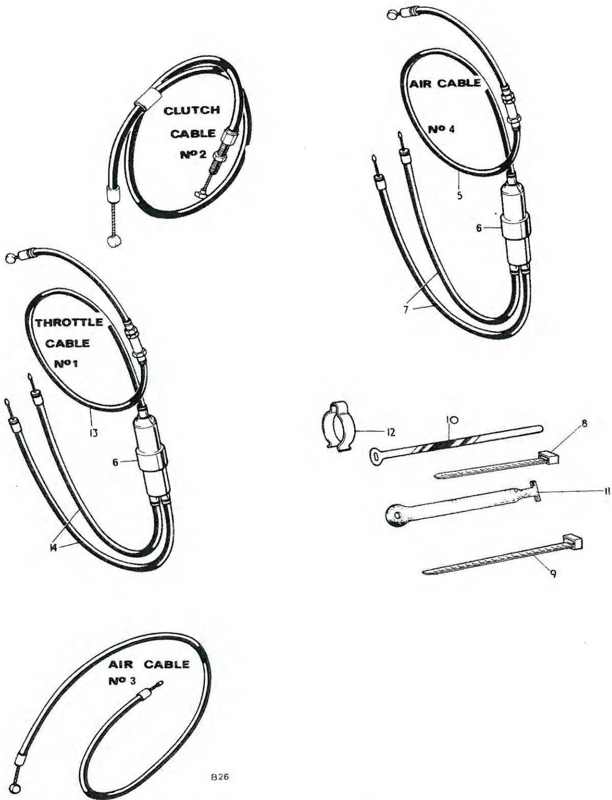
Fig. 30. CONTROL CABLES
