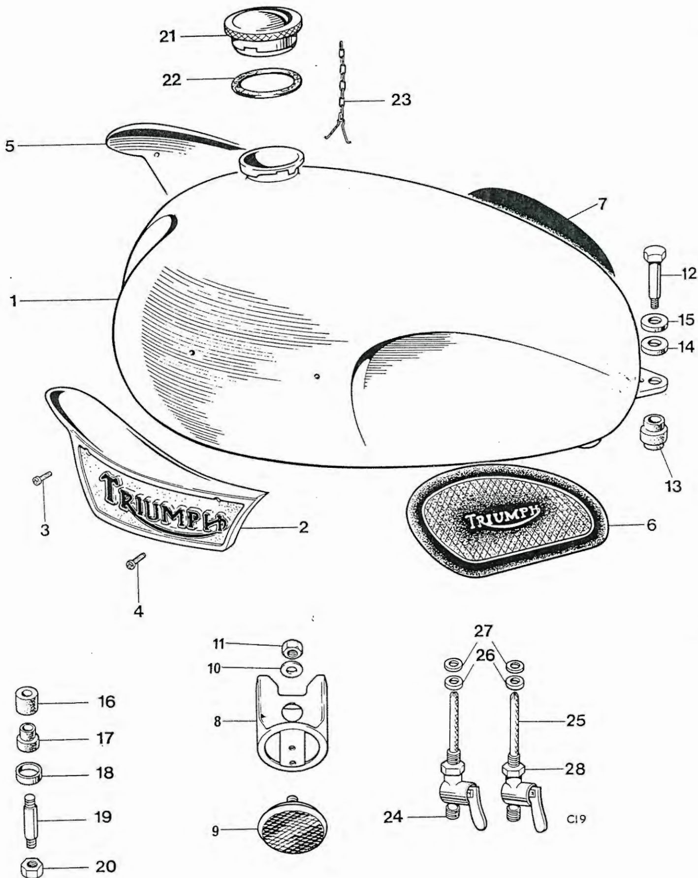
Fig. 22. GAS TANK
