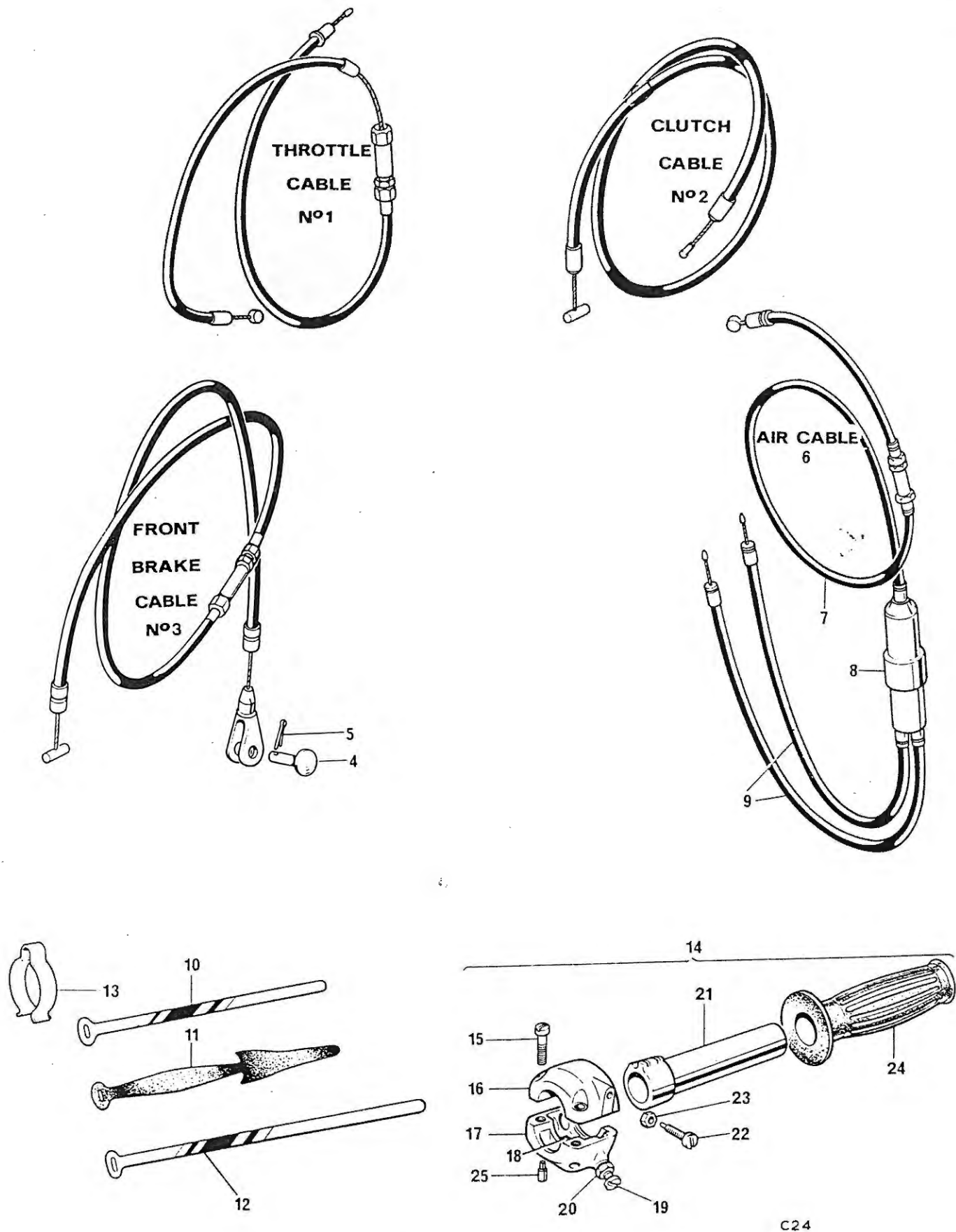
Fig. 26. CONTROL CABLES
