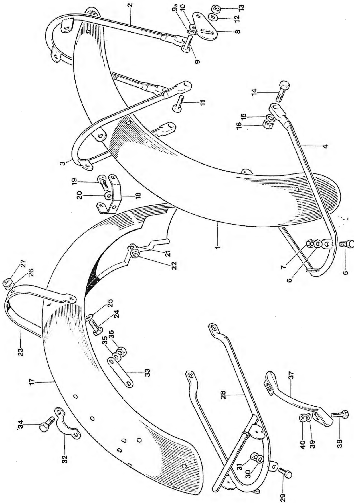
Fig. 19. FENDERS
