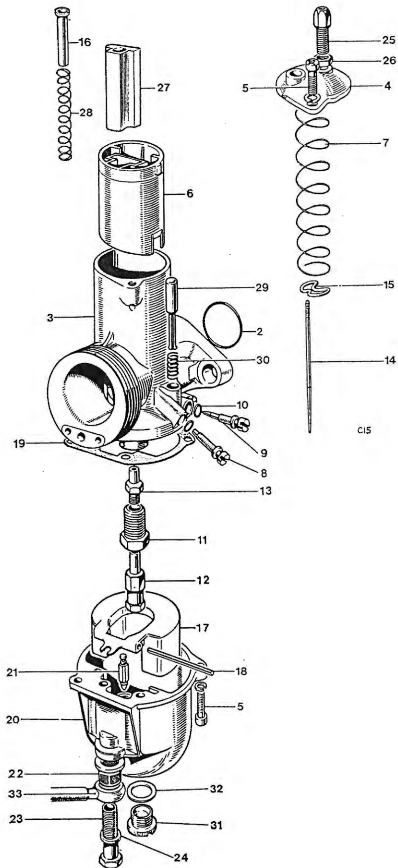
Fig. 5. CARBURETOR
