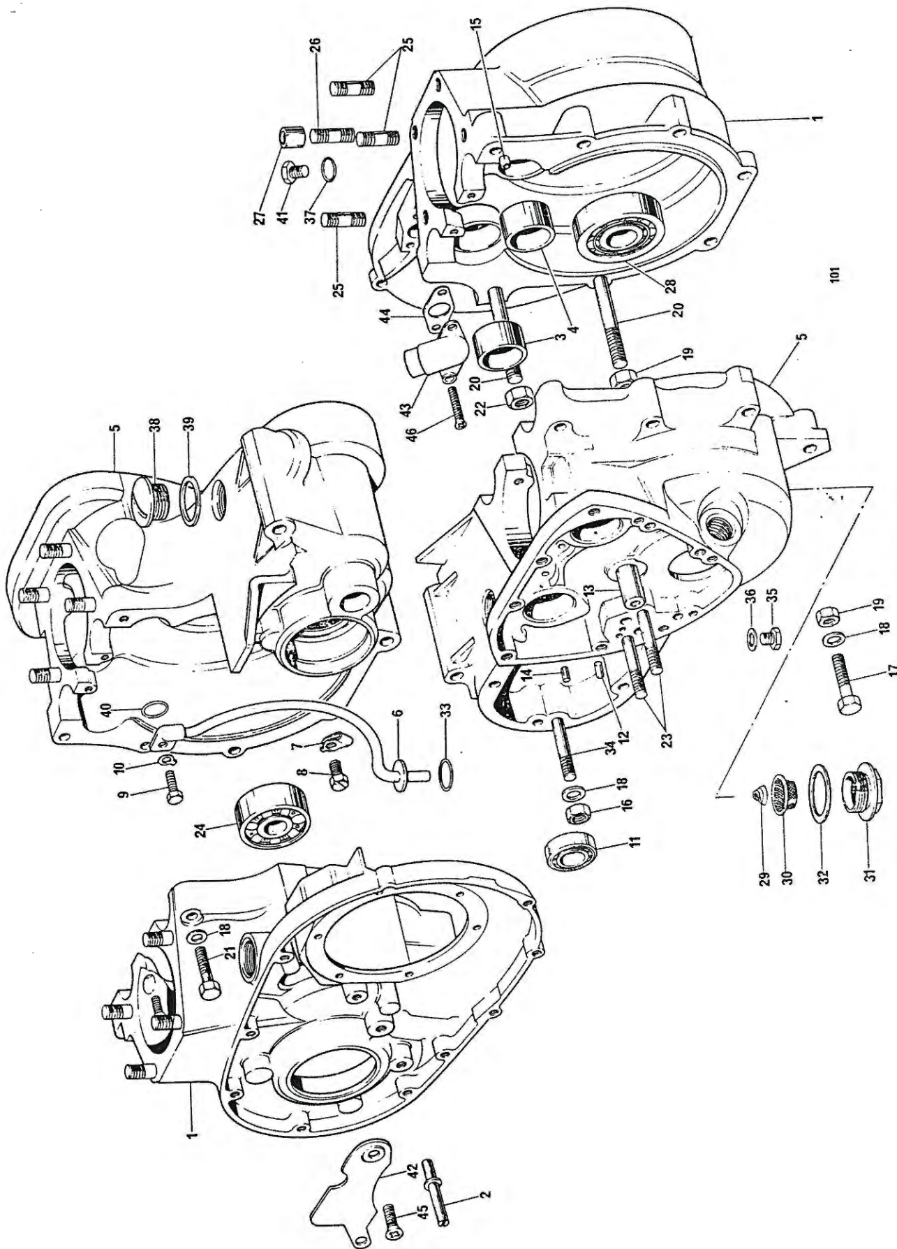
Fig. 2. CRANKCASE
