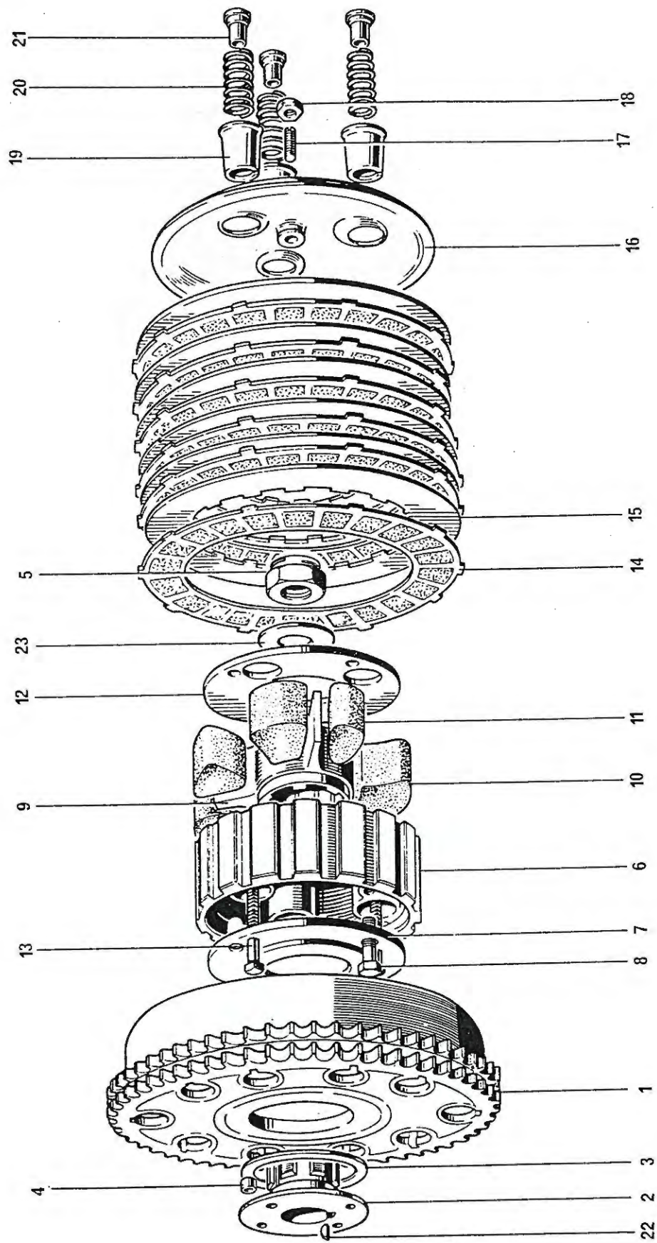
Fig. 10. CLUTCH
