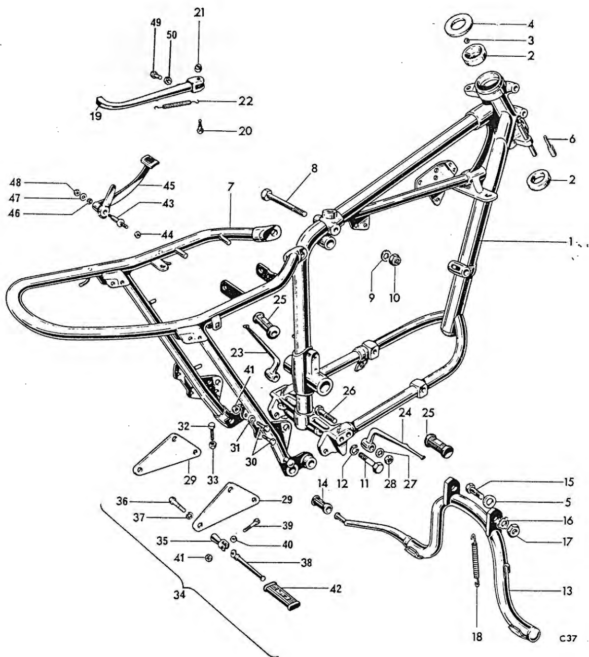
Fig. 14. FRAME
