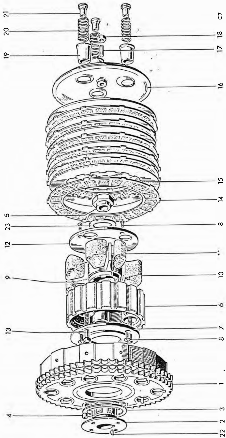
Fig. 13. CLUTCH
