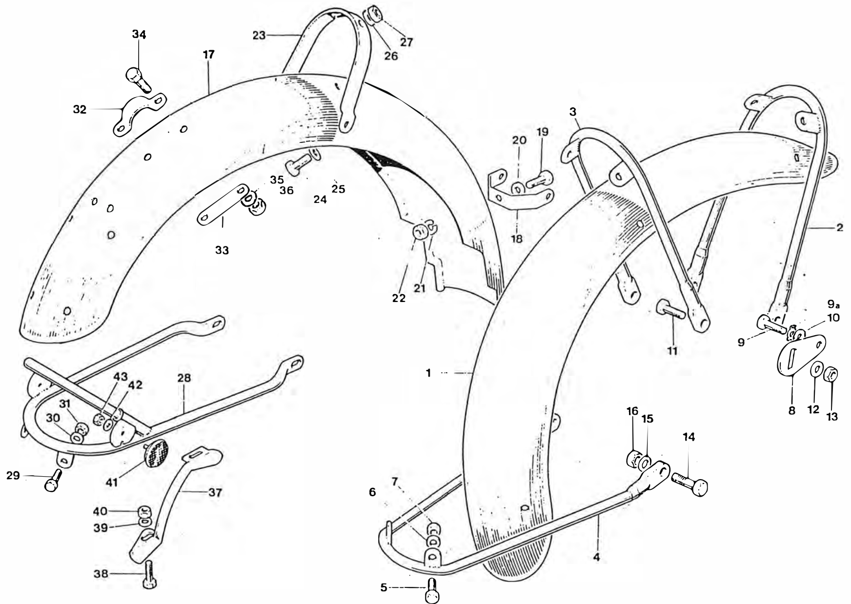
Fig. 24. FENDERS
