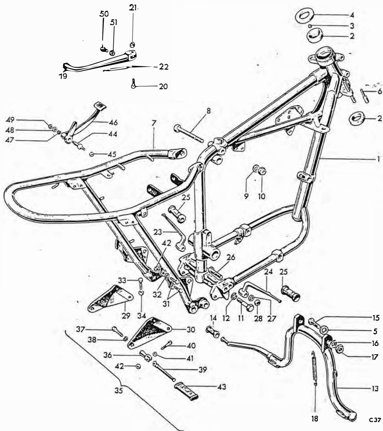
Fig. 18. FRAME
