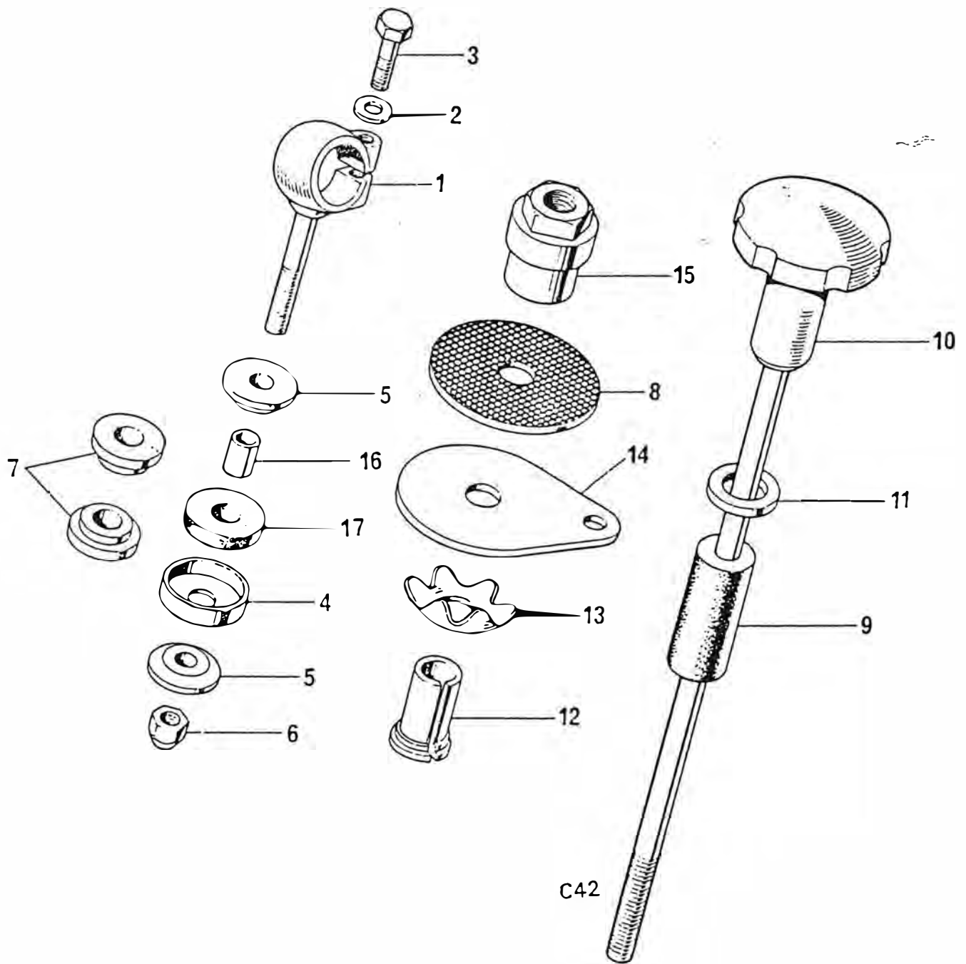
Fig. 30. STEERING DAMPER
